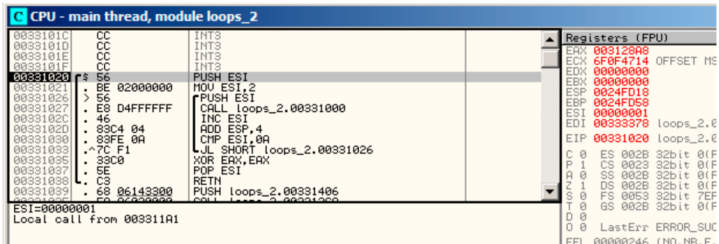
Рис. 1.46: OllyDbg: начало main()
