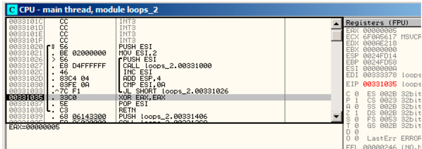
Рис. 1.48: OllyDbg: ESI = 10 , конец цикла
