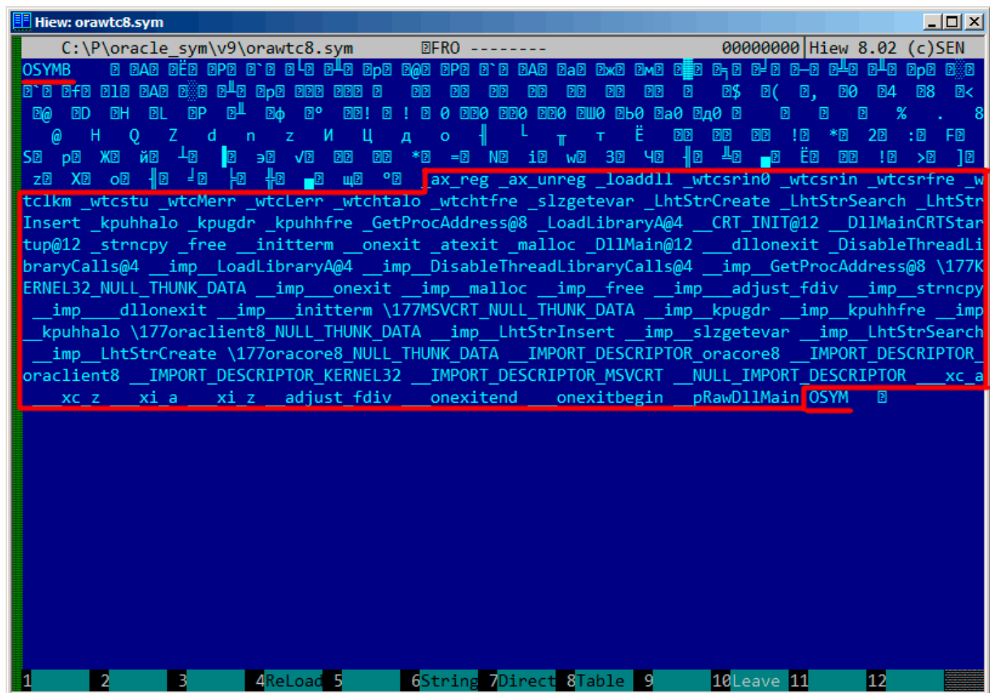
Рис. 9.22: Сигнатура OSYM и текстовые строки
