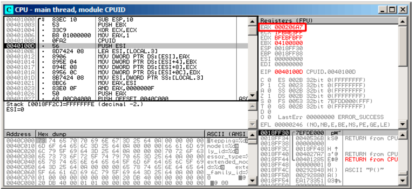
Рис. 1.100: OllyDbg: После исполнения CPUID
