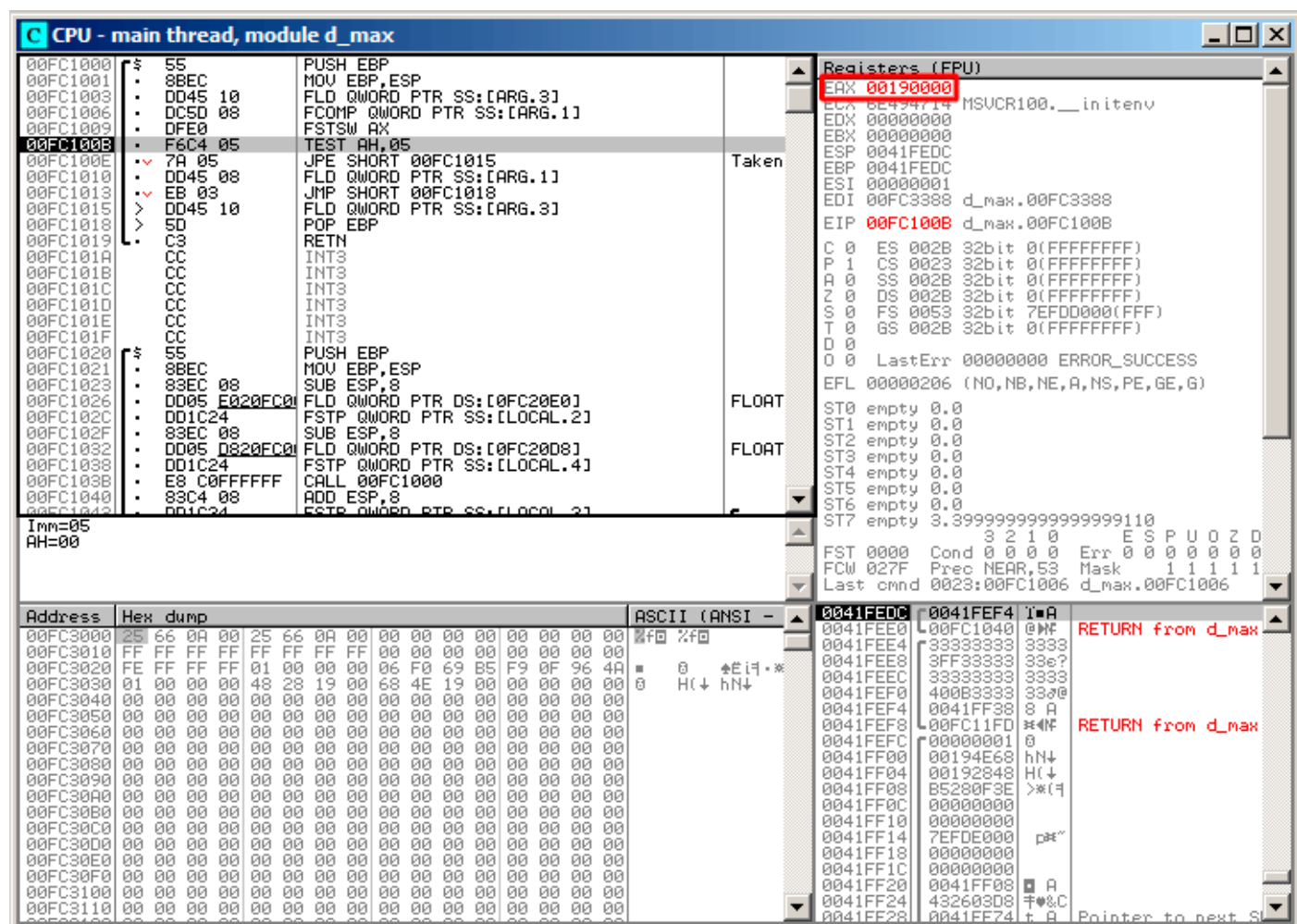
Рис. 1.61: OllyDbg: FNSTSW исполнилась
