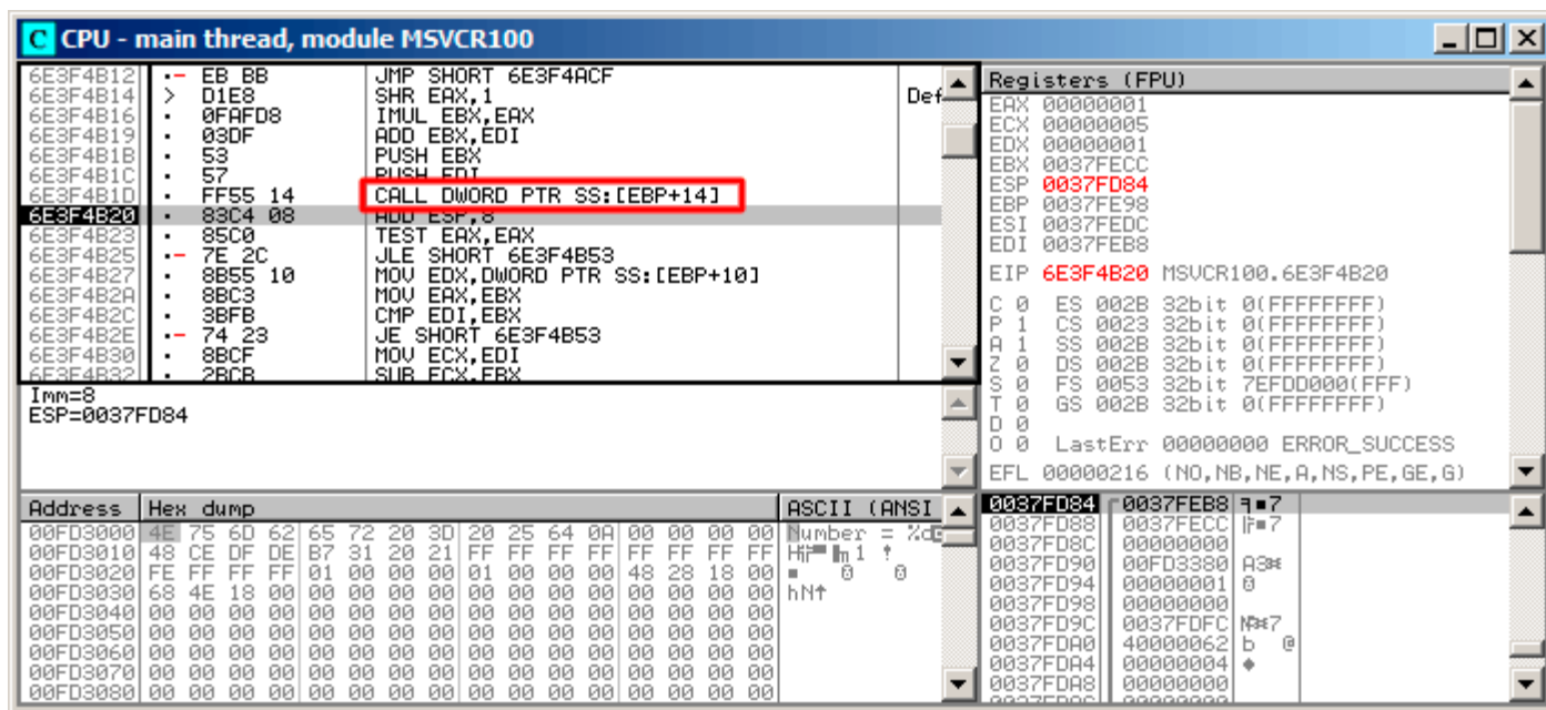
Рис. 1.102: OllyDbg: код в qsort() сразу после вызова comp()
