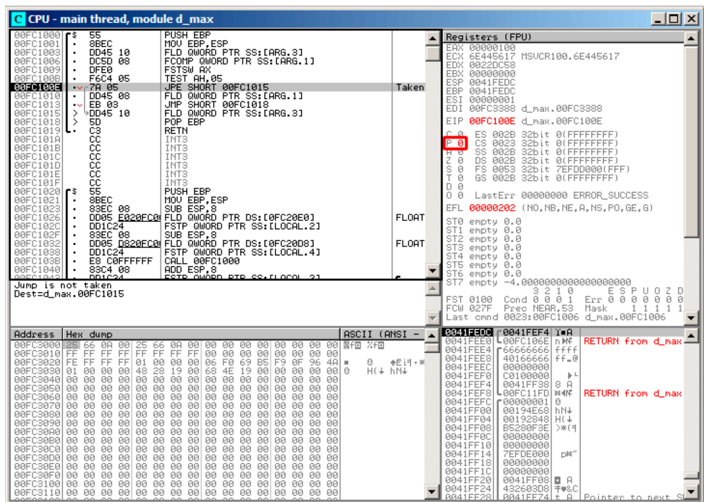
Рис. 1.67: OllyDbg: TEST исполнилась
