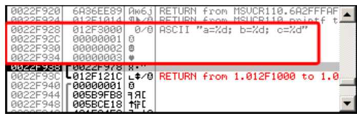
Рис. 1.9: OllyDbg: стек с сохраненными значениями (красная рамка добавлена в графическом редакторе)
