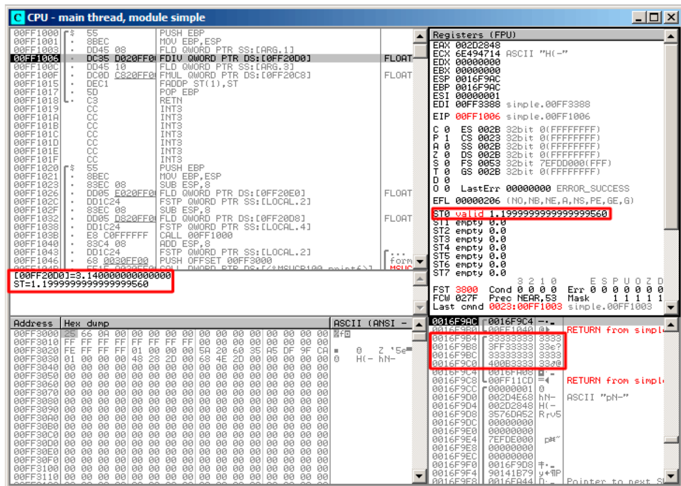
Рис. 1.54: OllyDbg: первая FLD исполнилась
