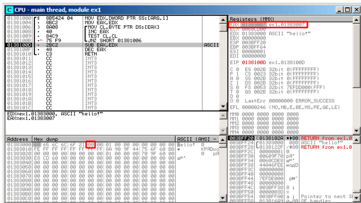
Рис. 1.52: OllyDbg: сейчас будет вычисление разницы указателей
