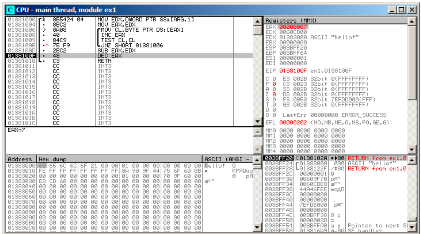
Рис. 1.53: OllyDbg: сейчас будет декремент EAX
