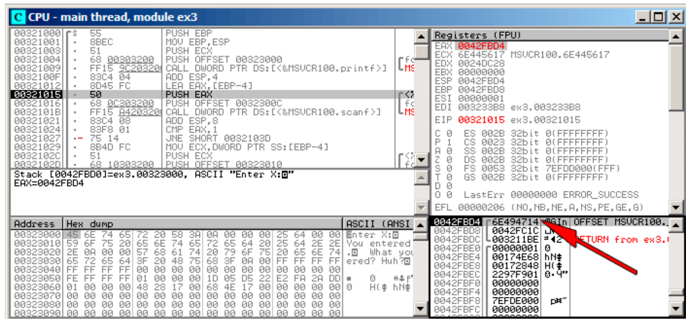
Рис. 1.19: OllyDbg: передача адреса переменной в scanf()
