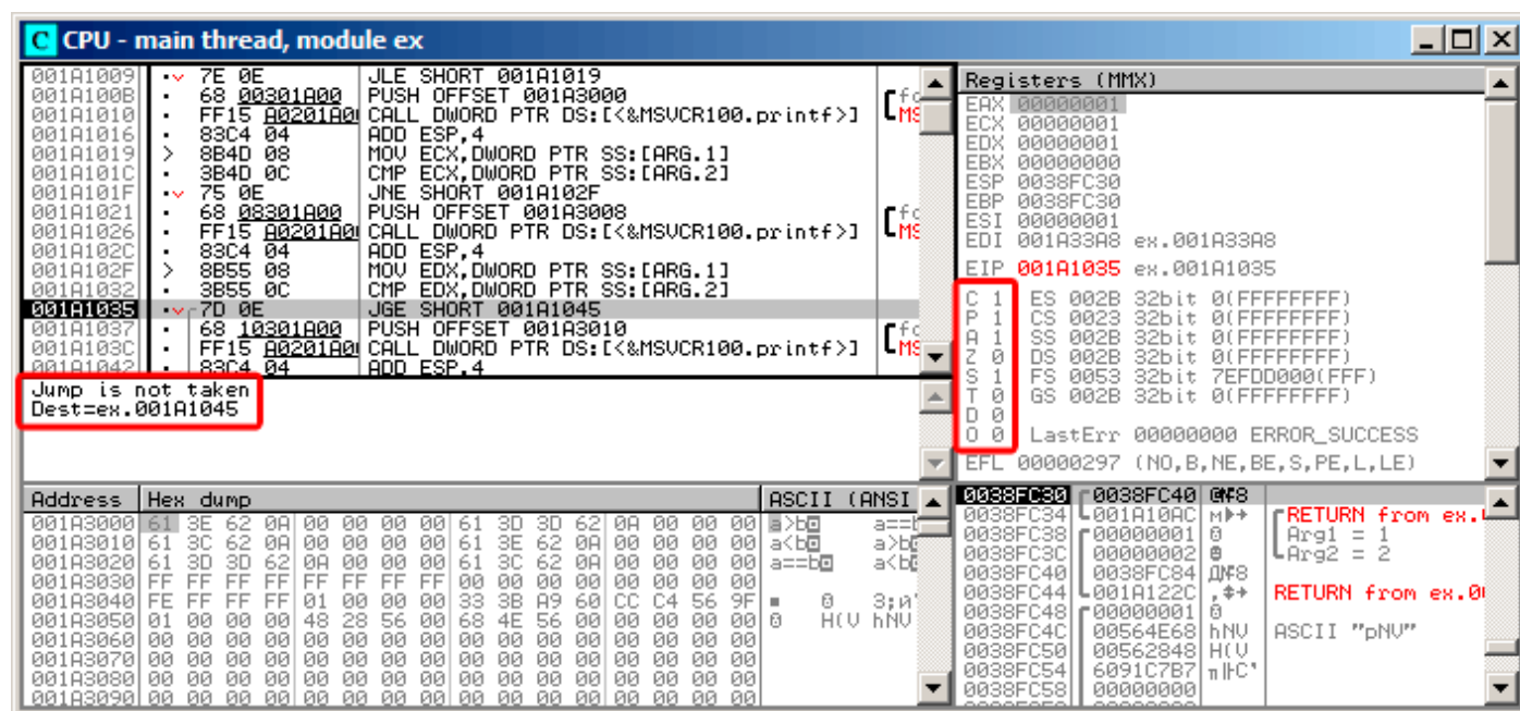
Рис. 1.31: OllyDbg: f_signed(): третий условный переход
