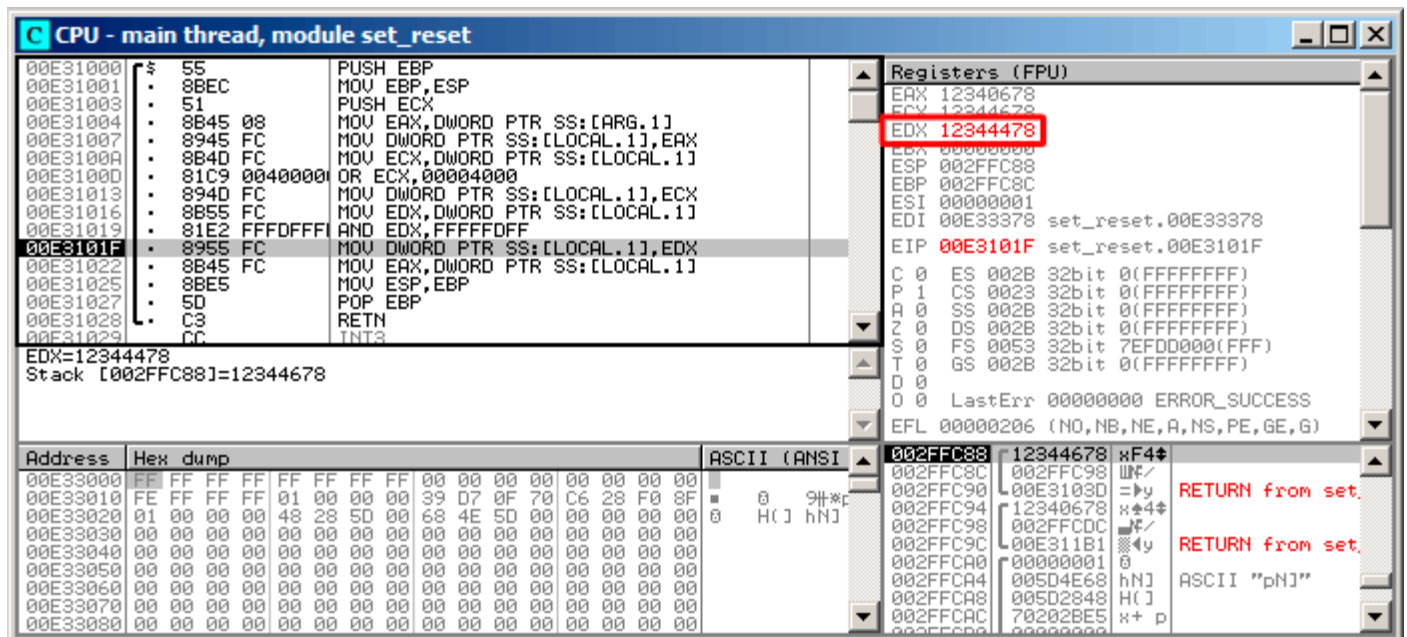
Рис. 1.89: OllyDbg: AND сработал
