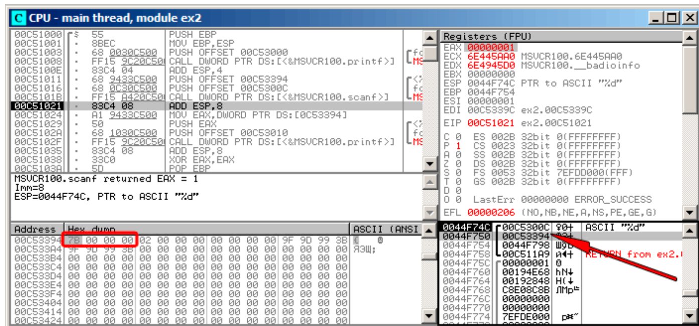
Рис. 1.15: OllyDbg: после исполнения scanf()
