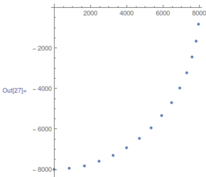
Рис. 8.12: Mathematica
