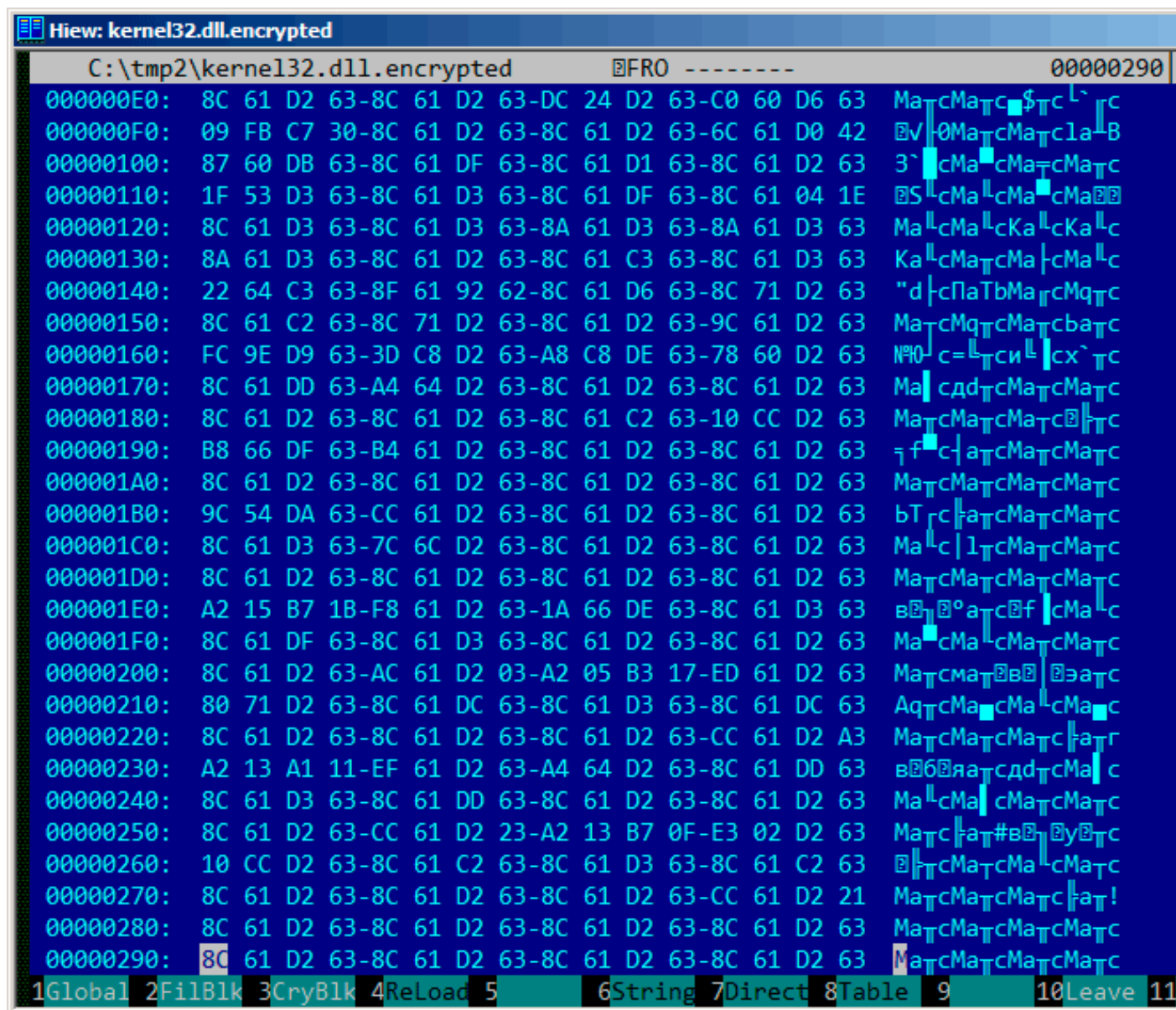
Рис. 9.6: «Зашифрованный» PE-заголовок
