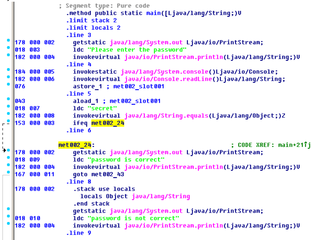
Рис. 4.5: IDA
