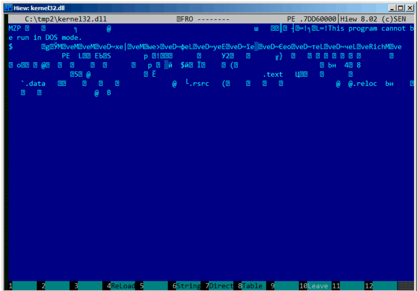
Рис. 9.3: Оригинальный файл
