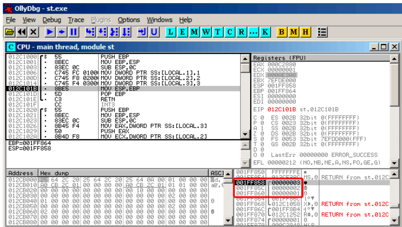
Рис. 1.5: OllyDbg: f1()
