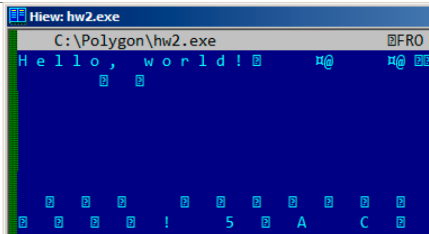
Рис. 5.3: Hiew
