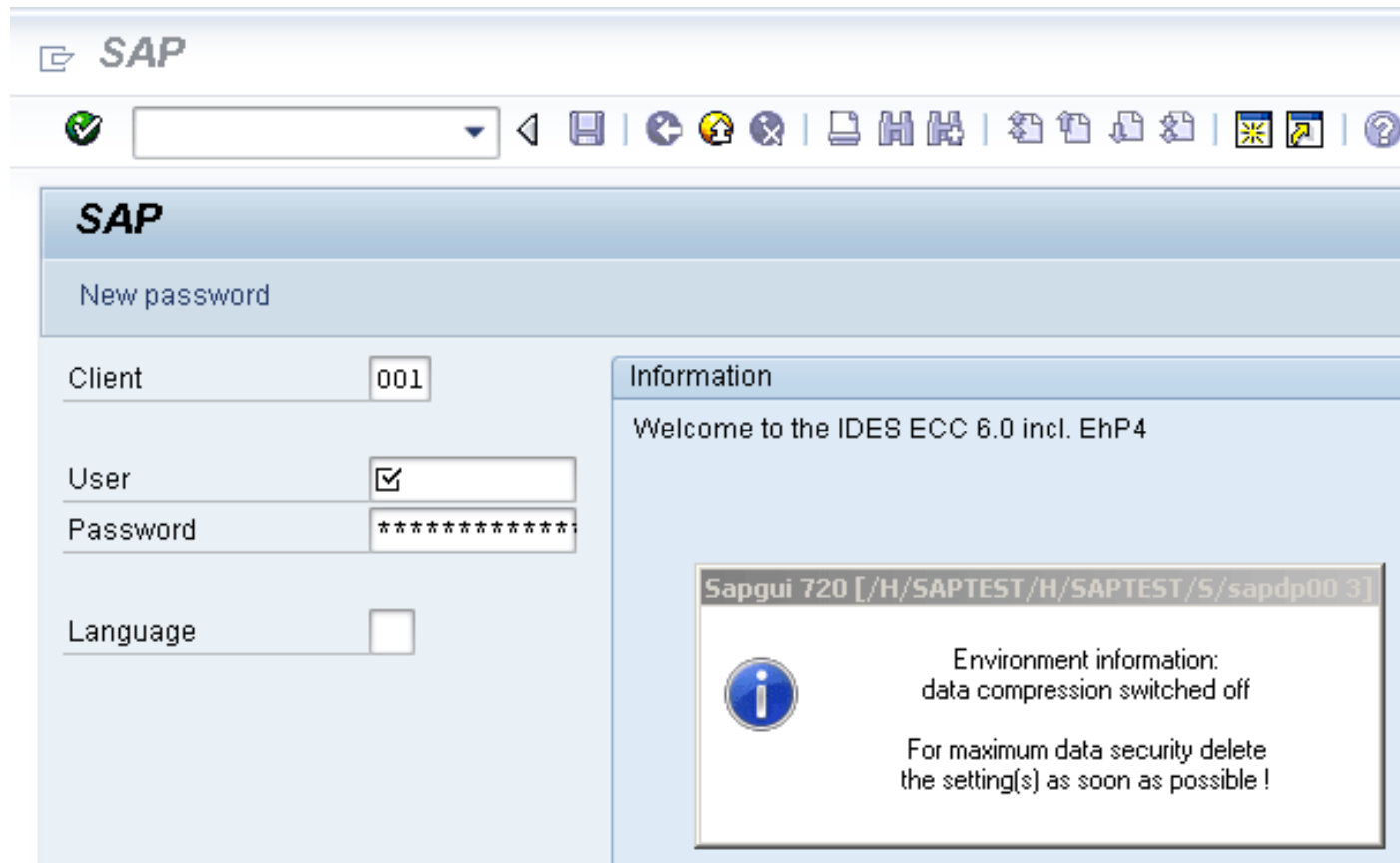
Рис. 8.15: Скриншот
