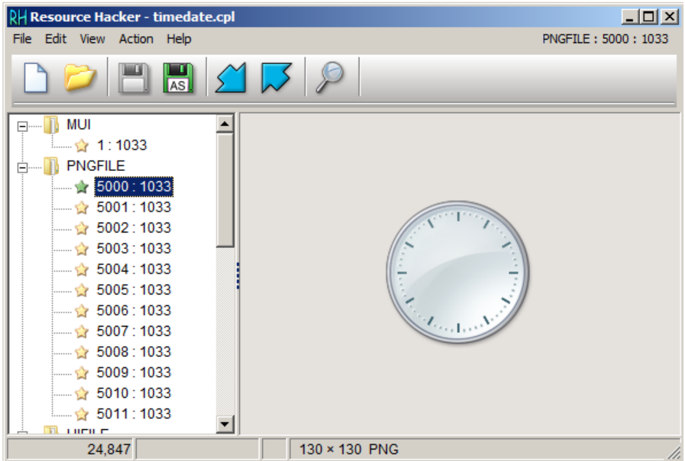
Рис. 8.10: Resource Hacker
