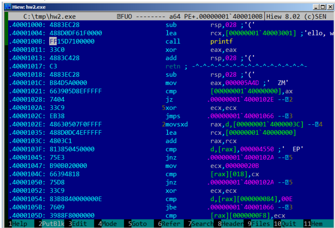
Рис. 1.4: Hiew
