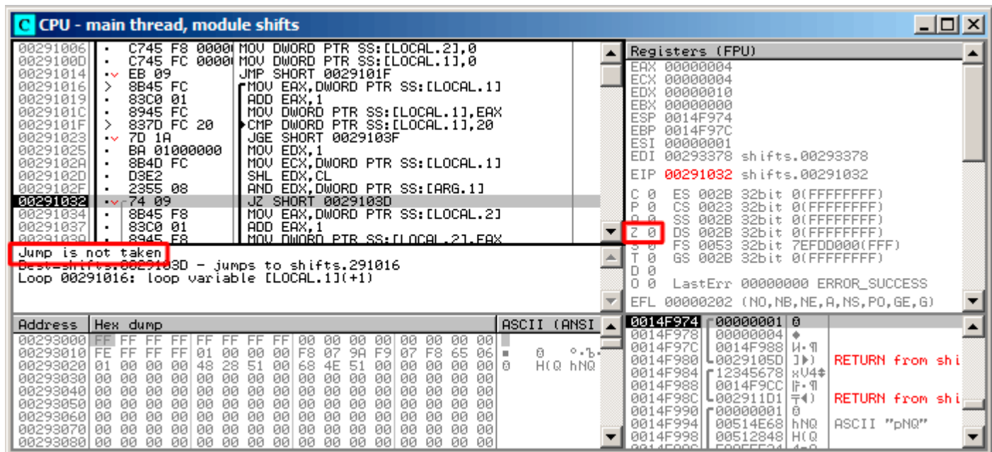
Рис. 1.95: OllyDbg: i = 4 , есть ли этот бит во входном значении? Да. (ZF = 0)
