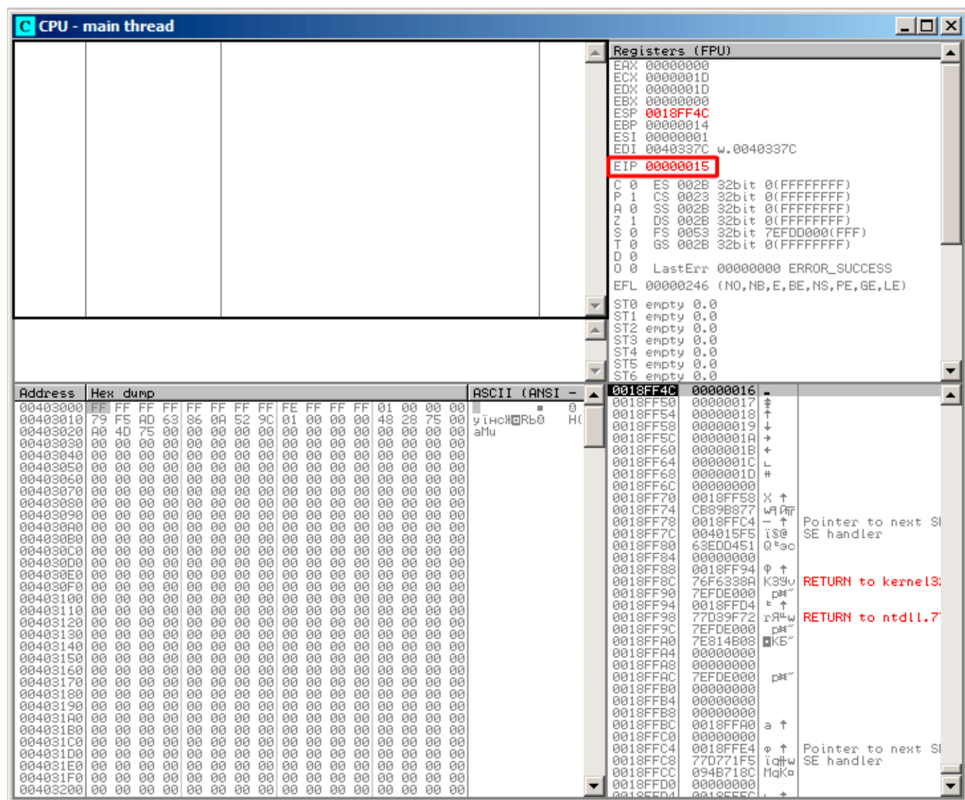
Рис. 1.83: OllyDbg: EIP восстановлен, но OllyDbg не может дизассемблировать по адресу 0x15
