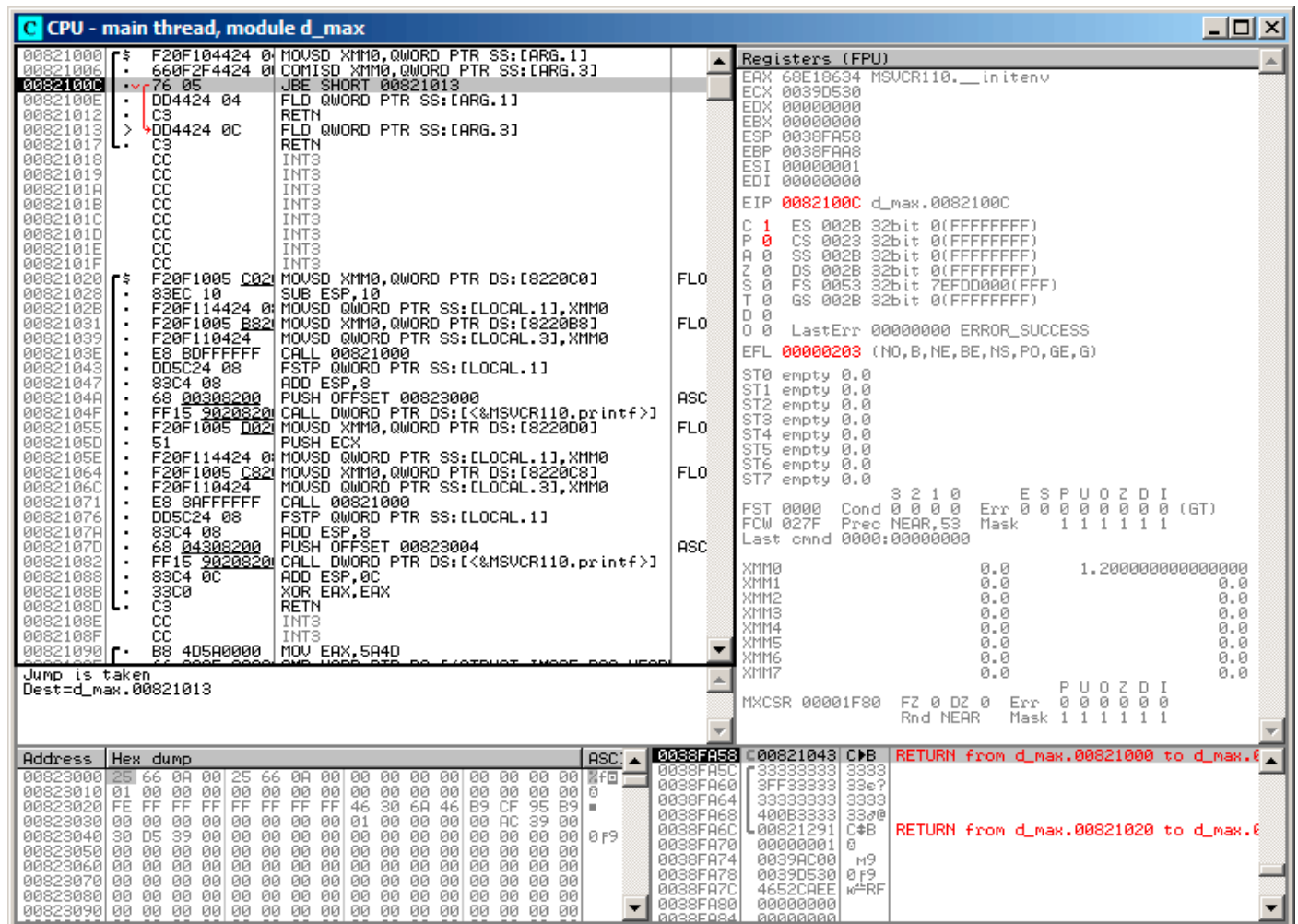
Рис. 1.110: OllyDbg: COMISD изменила флаги CF и PF
