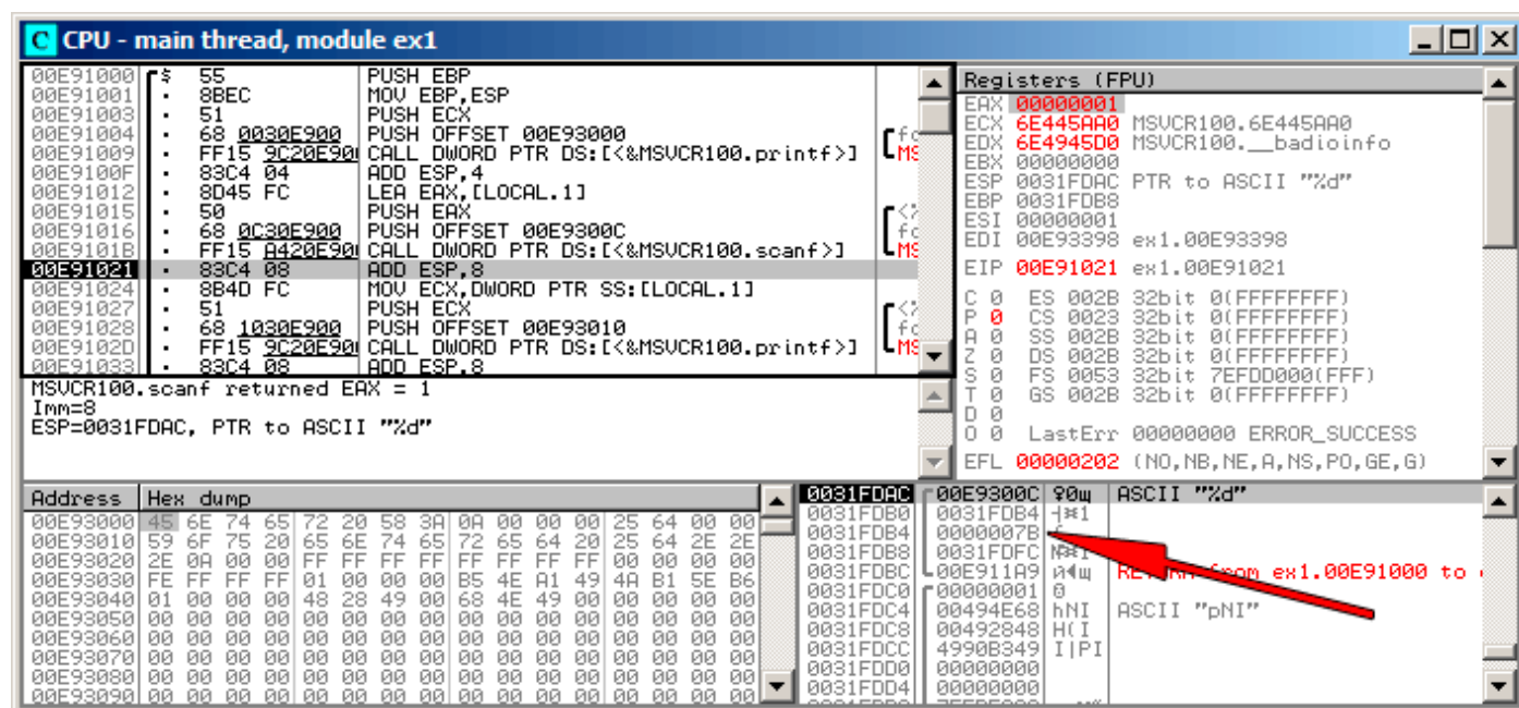
Рис. 1.13: OllyDbg: scanf() исполнилась
