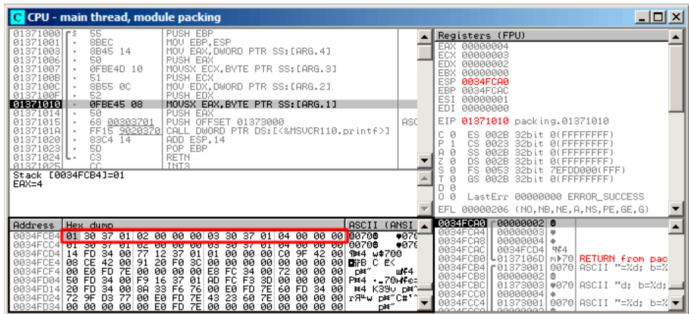
Рис. 1.97: OllyDbg: Перед исполнением printf()
