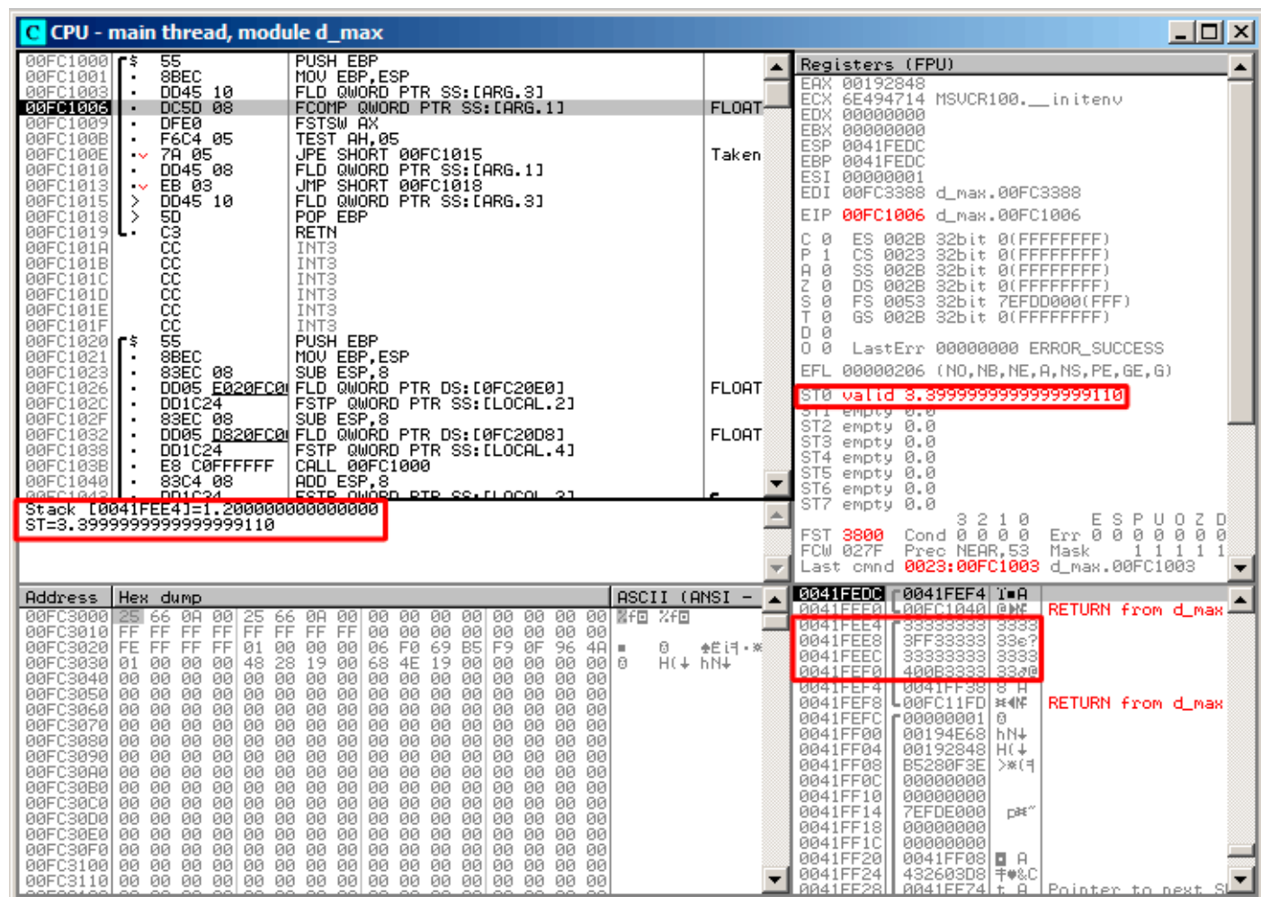
Рис. 1.59: OllyDbg: первая FLD исполнилась
