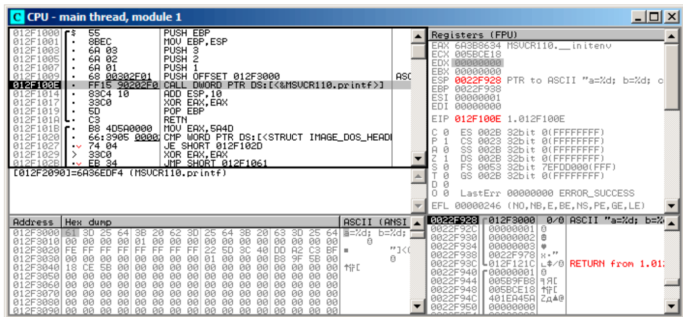
Рис. 1.8: OllyDbg: перед исполнением printf()
