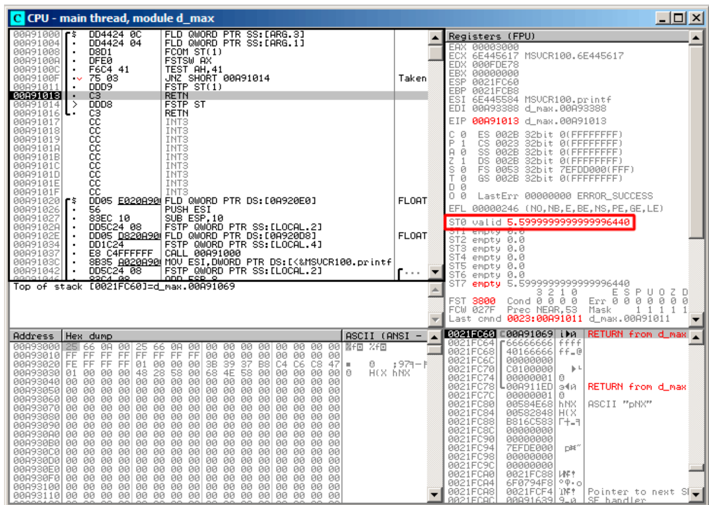
Рис. 1.78: OllyDbg: FSTP исполнилась
