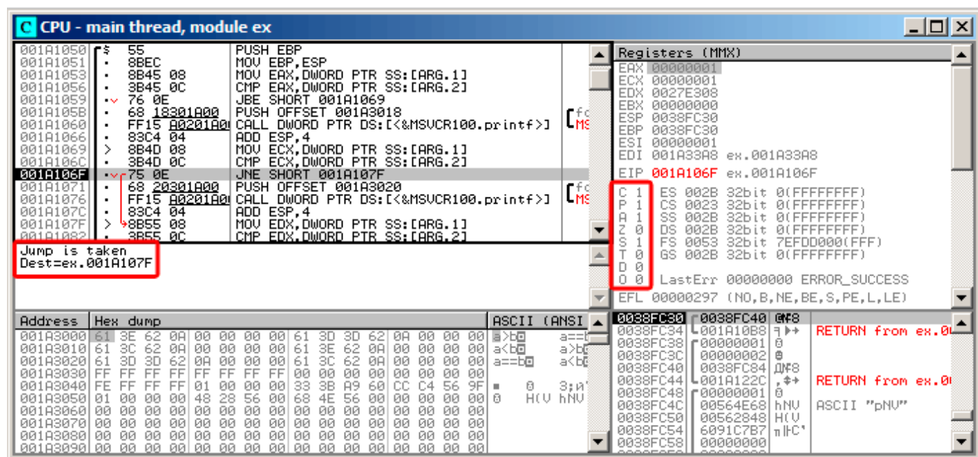
Рис. 1.27: OllyDbg: f_unsigned(): второй условный переход
