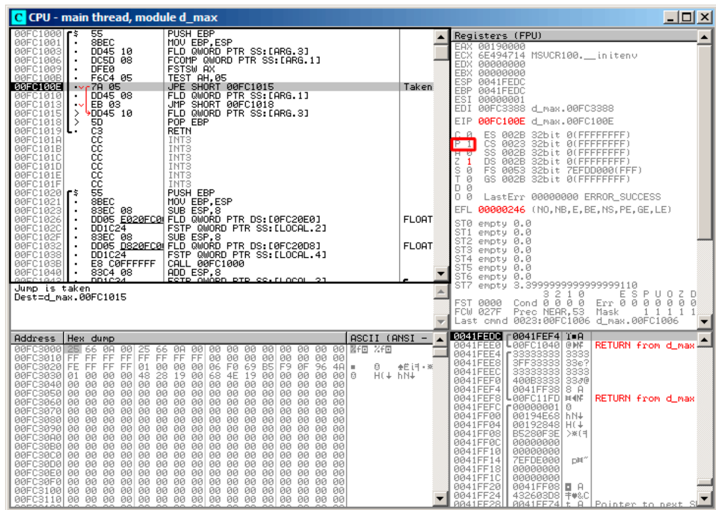
Рис. 1.62: OllyDbg: TEST исполнилась
