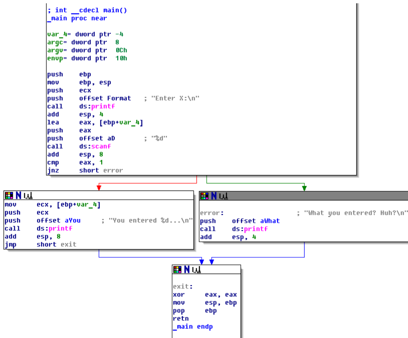
Рис. 1.17: Отображение функции в IDA в виде графа
