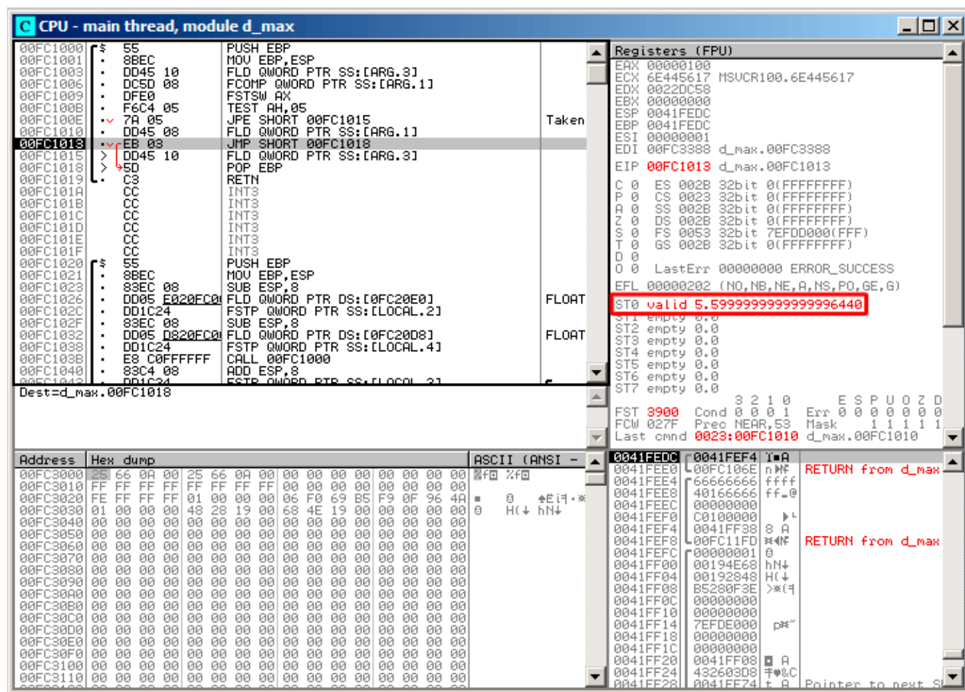
Рис. 1.68: OllyDbg: вторая FLD исполнилась
