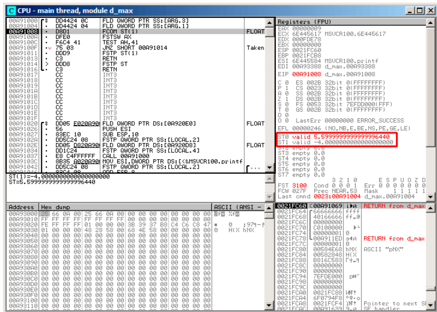
Рис. 1.74: OllyDbg: обе FLD исполнились
