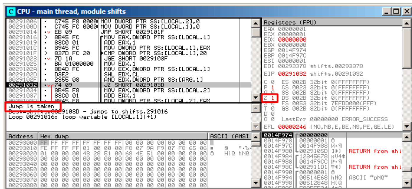
Рис. 1.92: OllyDbg: i = 1 , есть ли этот бит во входном значении? Нет. (ZF = 1)
