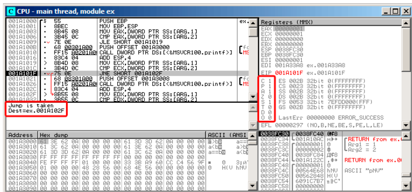
Рис. 1.30: OllyDbg: f_signed(): второй условный переход
