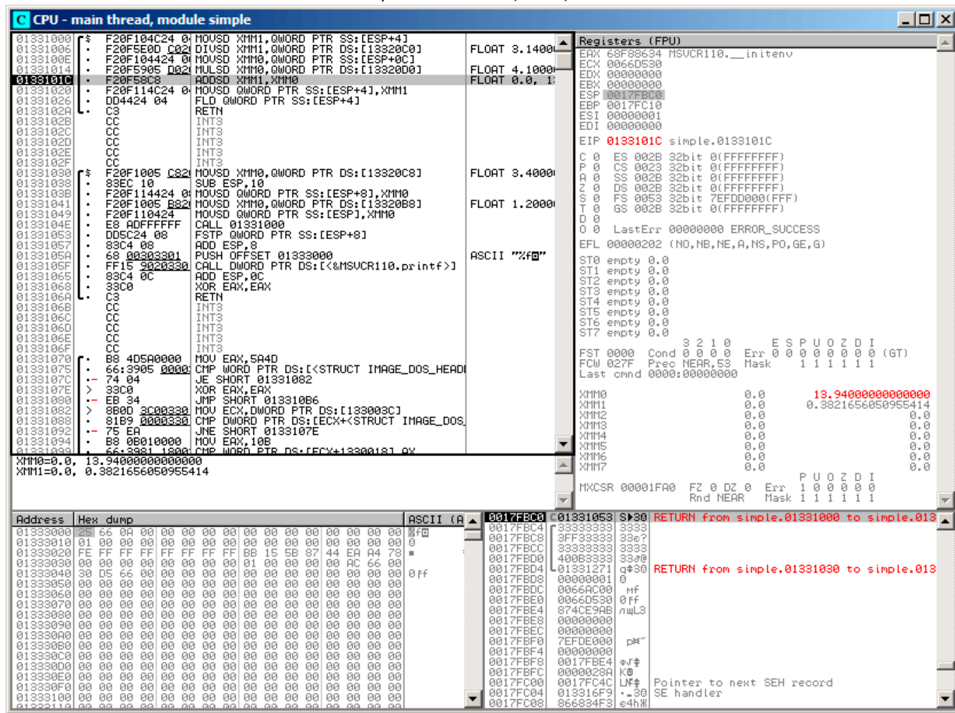
Рис. 1.107: OllyDbg: MULSD вычислила product и оставила его в XMM0
