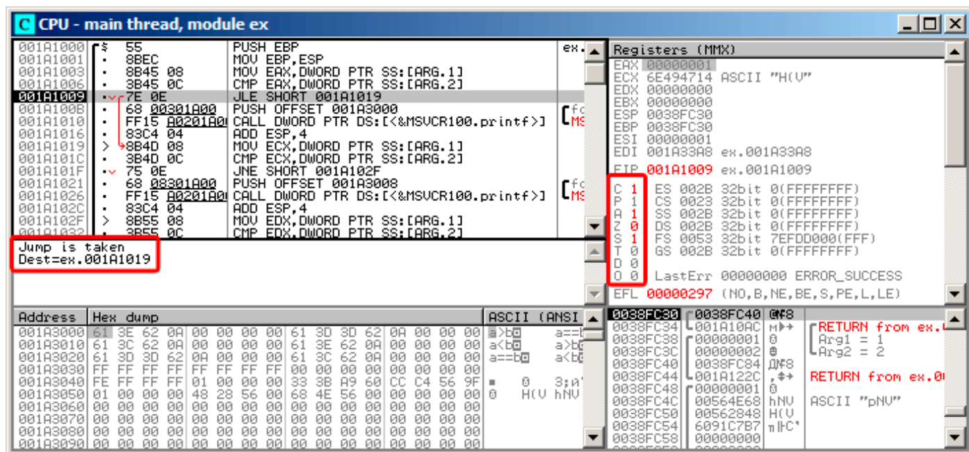
Рис. 1.29: OllyDbg: f_signed() : первый условный переход
