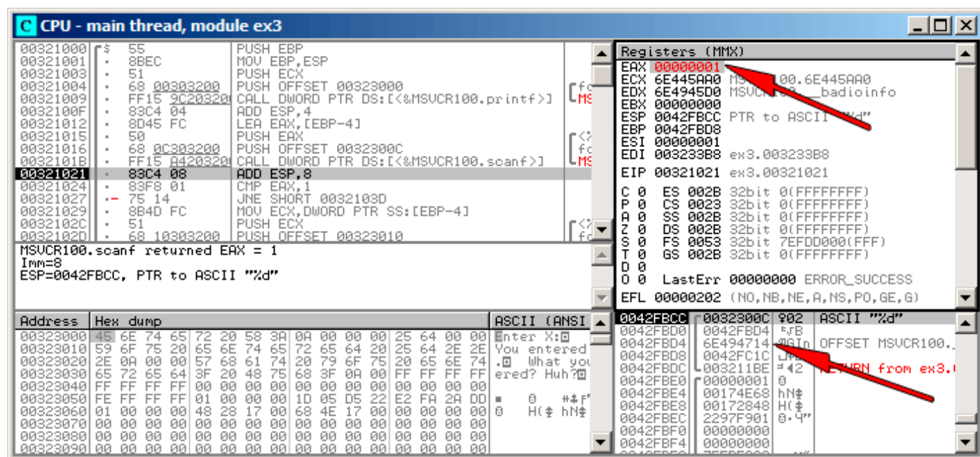
Рис. 1.20: OllyDbg: scanf() закончился с ошибкой
