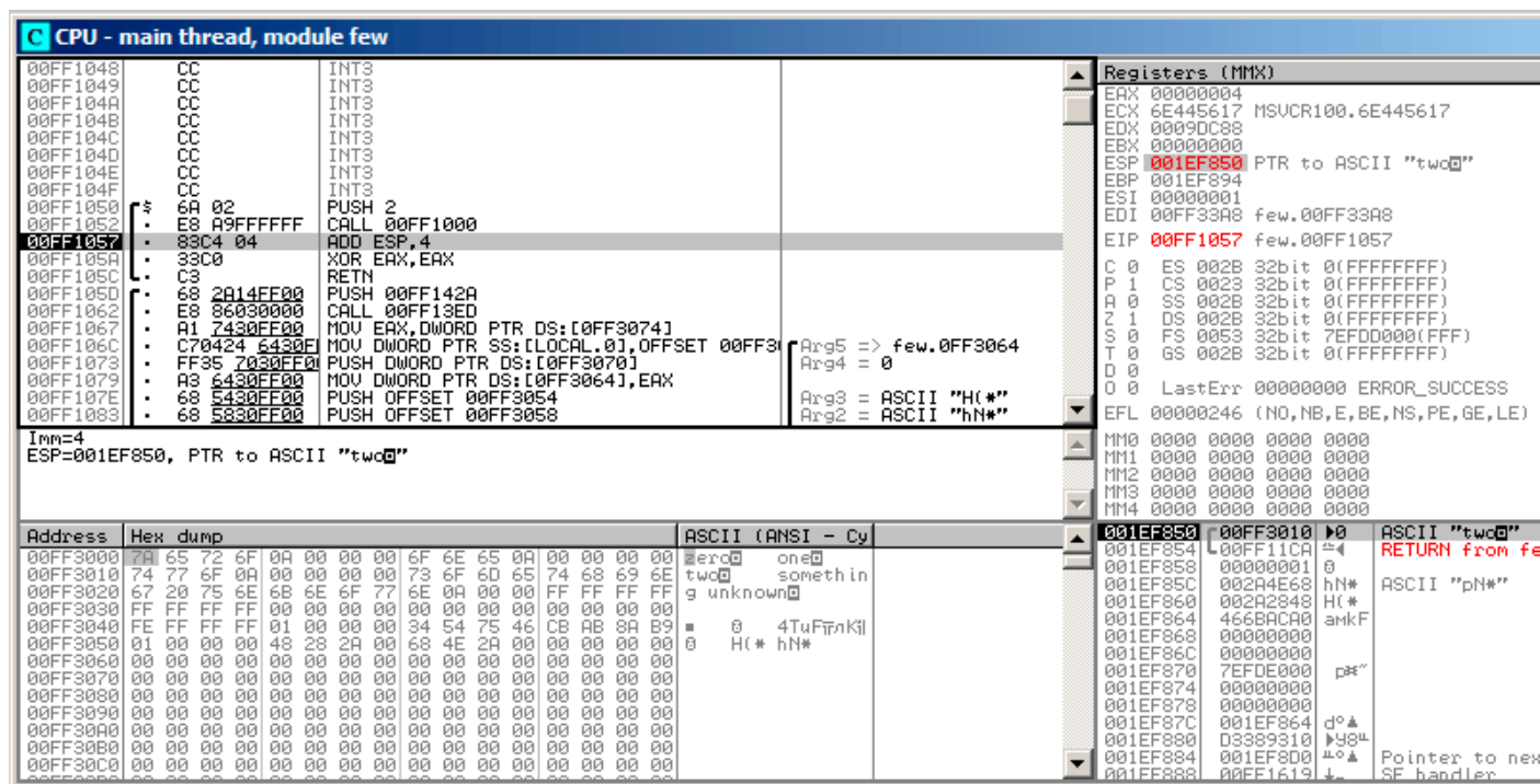
Рис. 1.41: OllyDbg: возврат в main()
