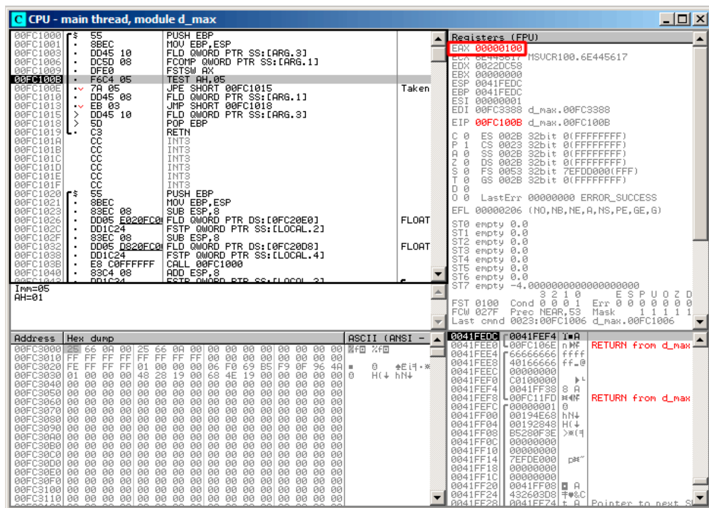
Рис. 1.66: OllyDbg: FNSTSW исполнилась
