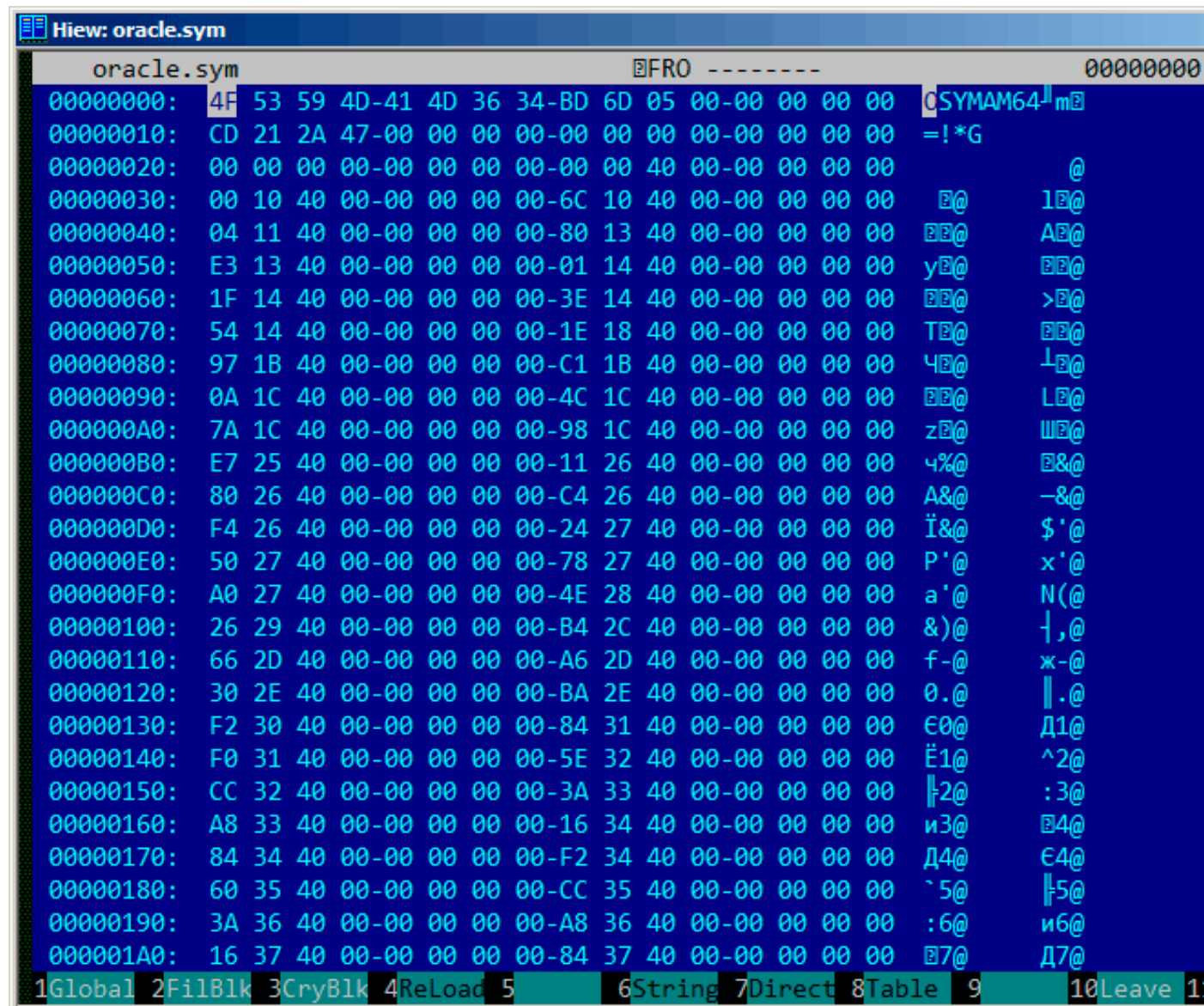
Рис. 9.25: пример .SYM-файла из Oracle RDBMS для win64
