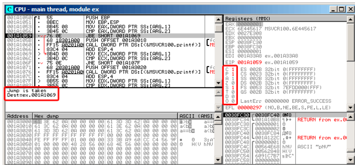
Рис. 1.26: OllyDbg: f_unsigned() : первый условный переход
