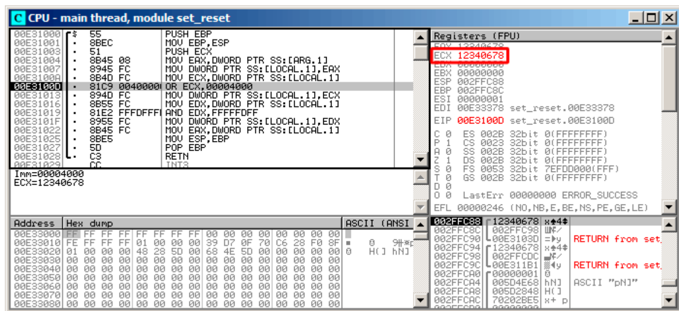
Рис. 1.86: OllyDbg: значение загружено в ECX
