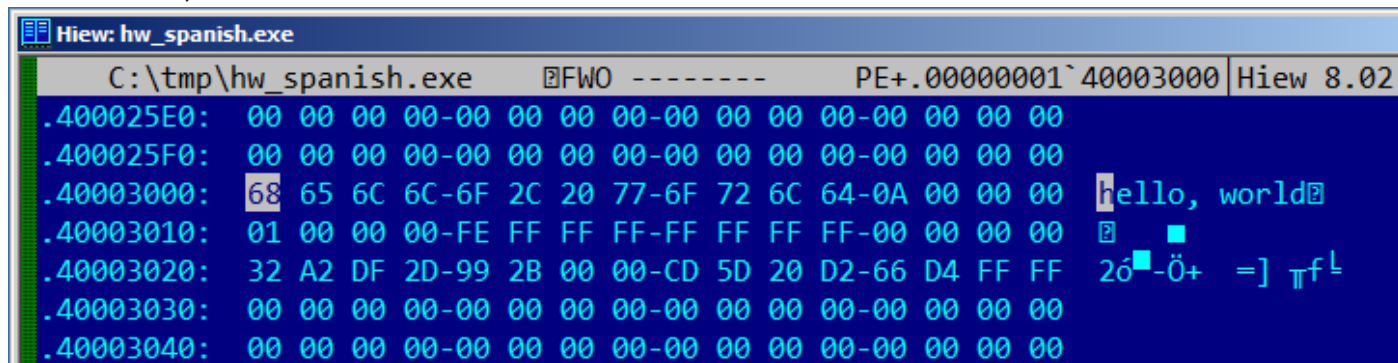
Рис. 1.1: Hiew
