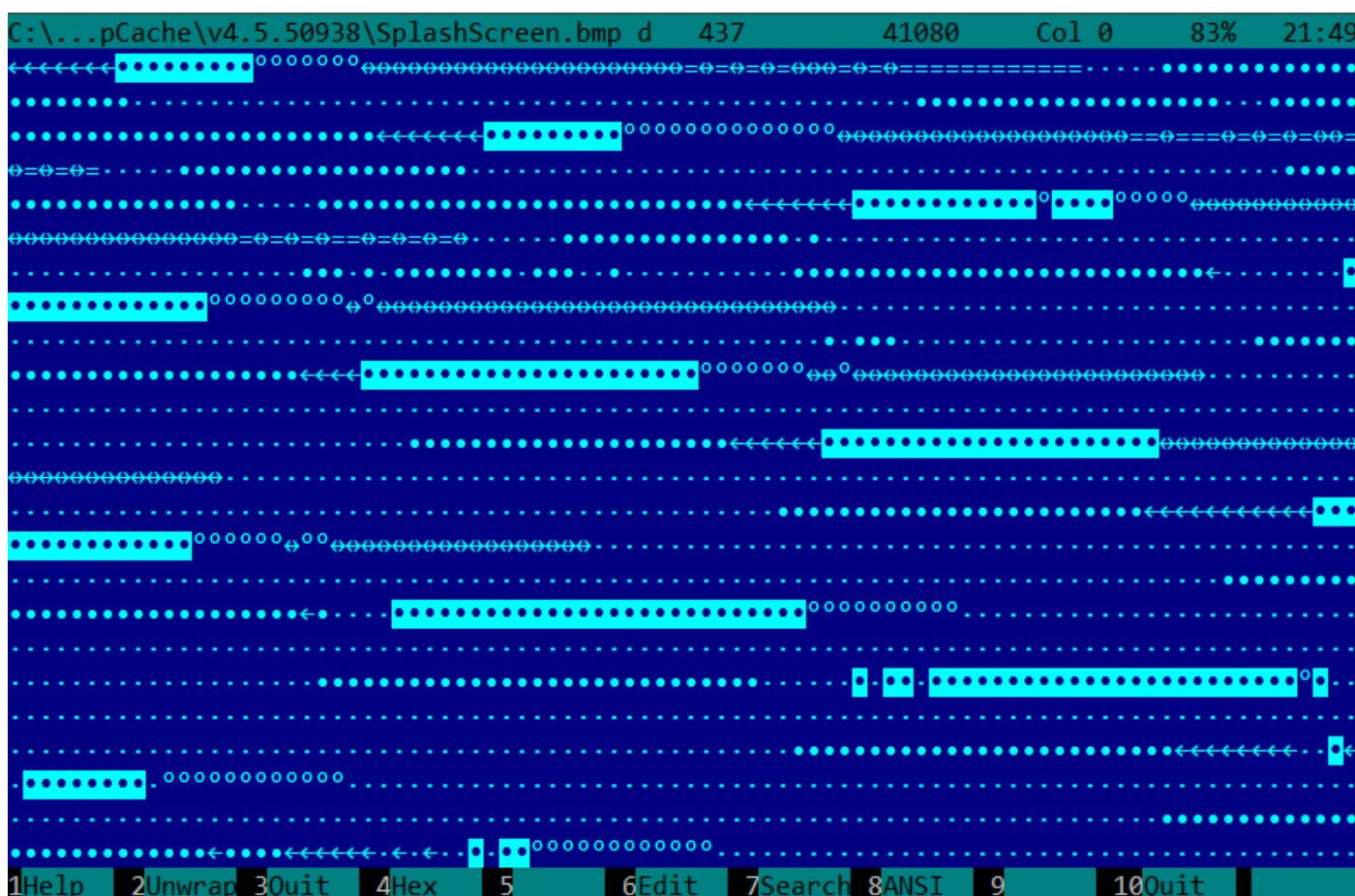
Рис. 5.15: Фрагмент BMP-файла
