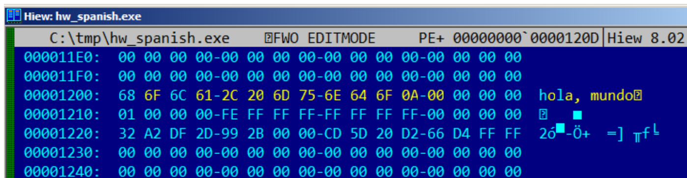
Рис. 1.2: Hiew
