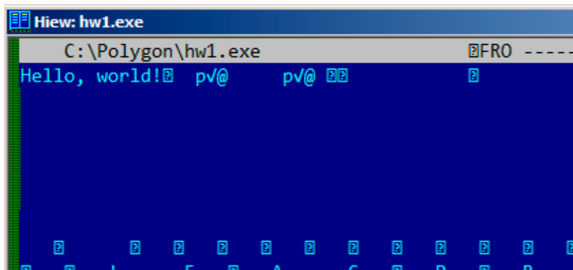
Рис. 5.1: Hiew
