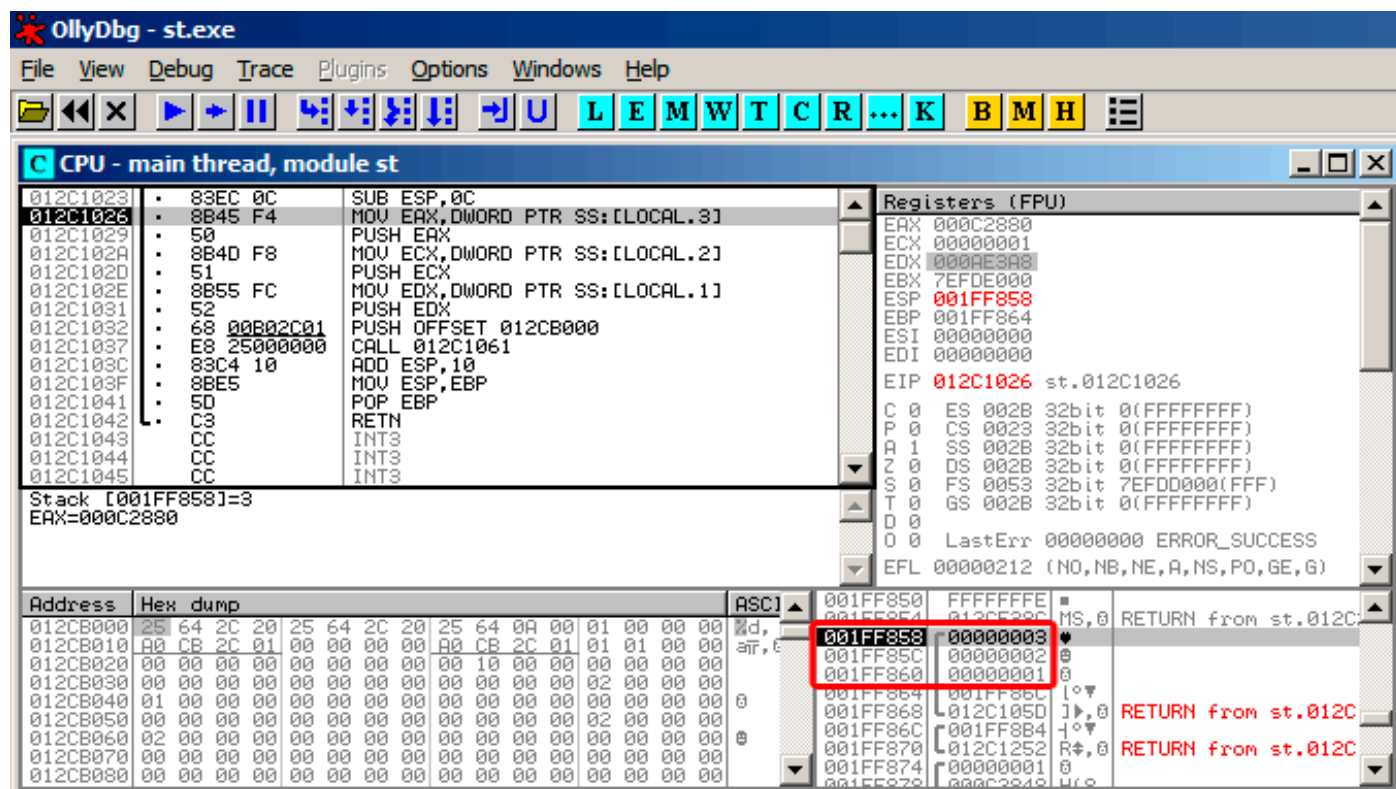
Рис. 1.6: OllyDbg: f2()
