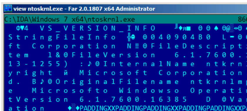
Рис. 5.4: Hiew
