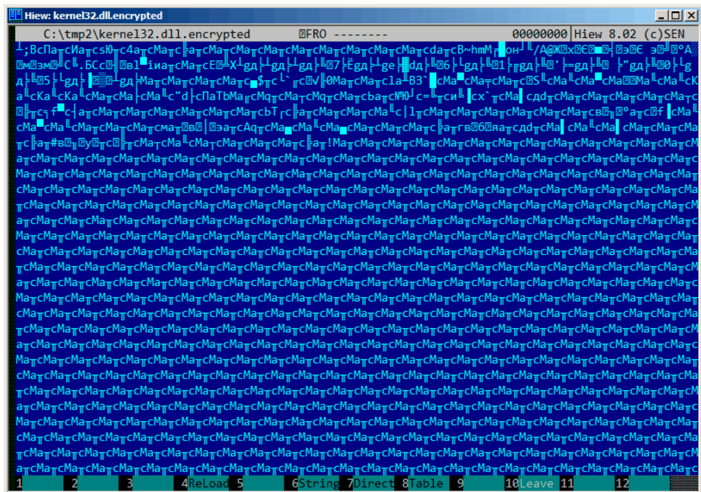
Рис. 9.4: «Зашифрованный» файл
