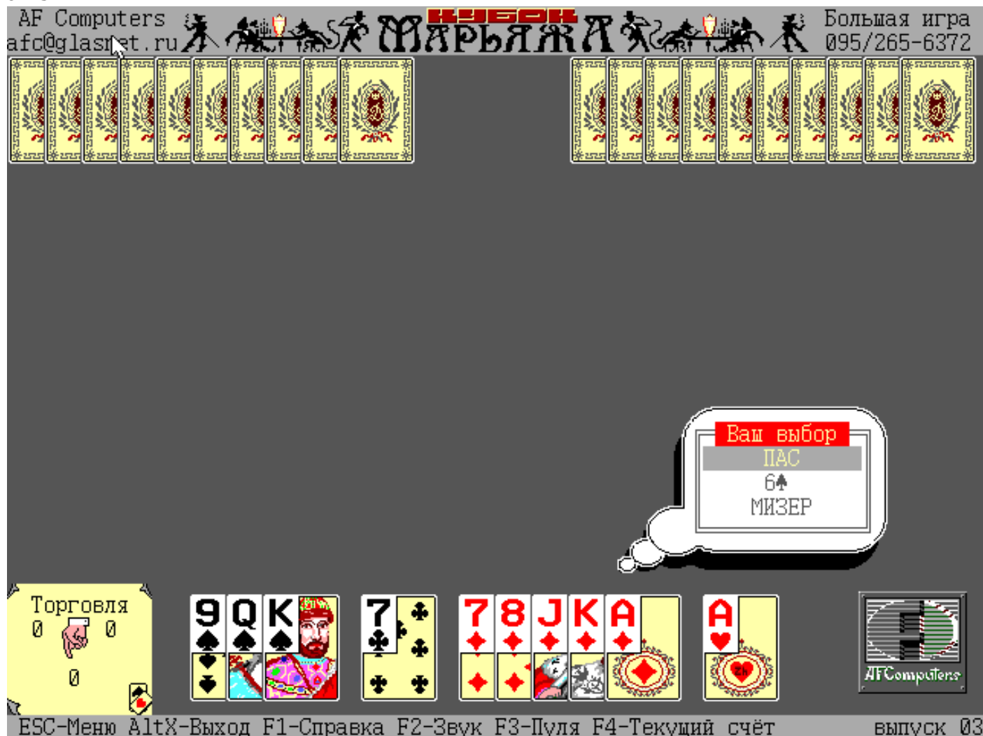
Рис. 8.22: "Прикупа" нет
