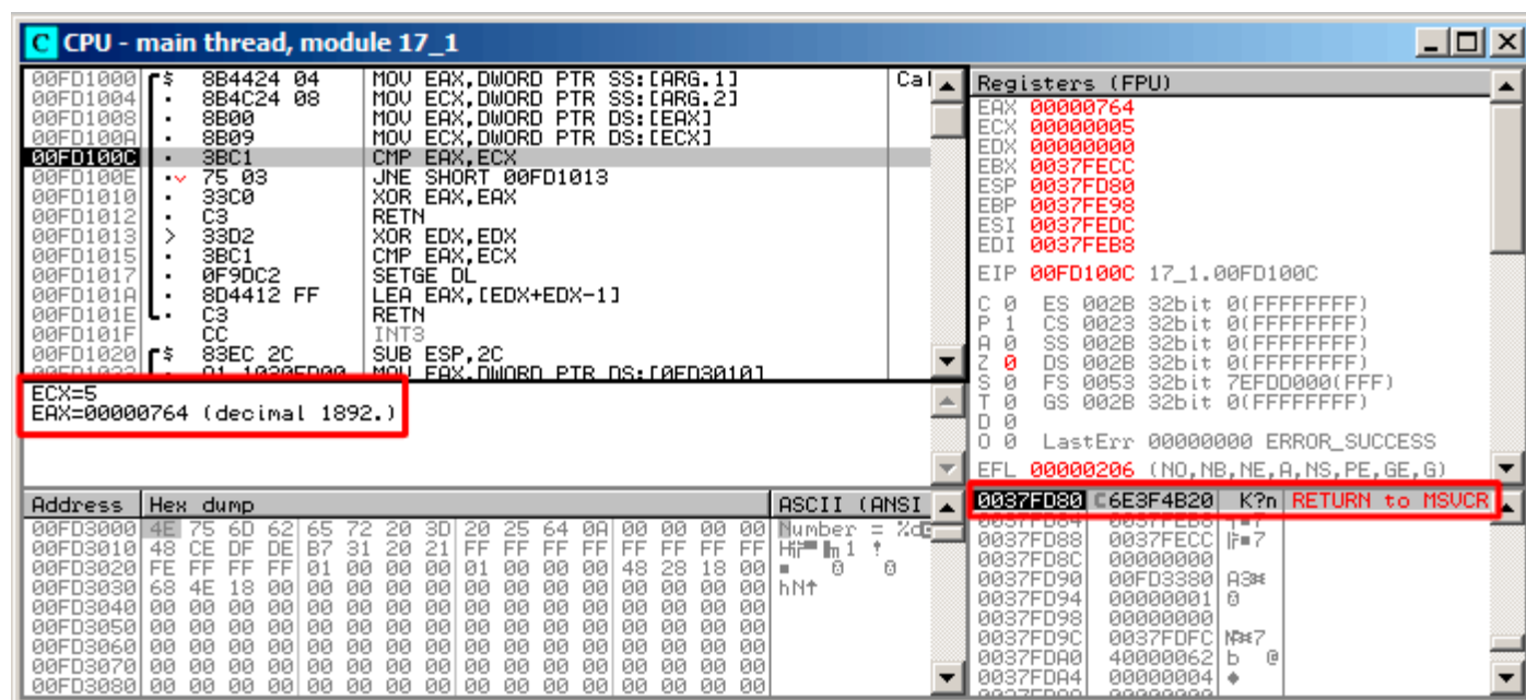
Рис. 1.101: OllyDbg: первый вызов comp()
