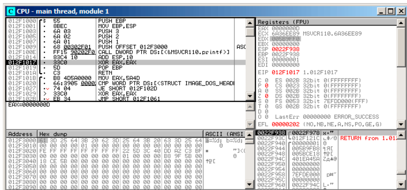
Рис. 1.11: OllyDbg: после исполнения инструкции ADD ESP, 10
