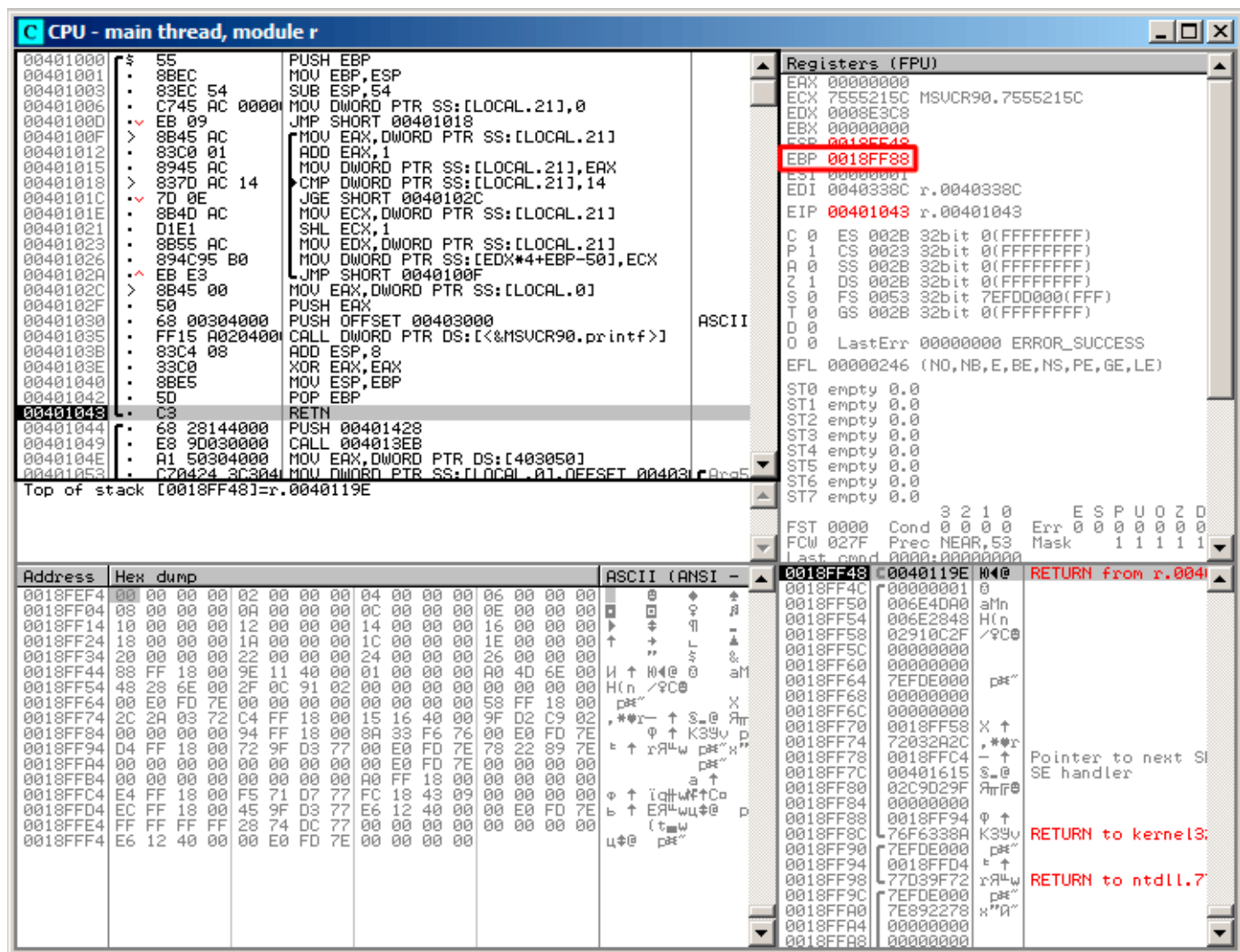
Рис. 1.81: OllyDbg: восстановление EBP
