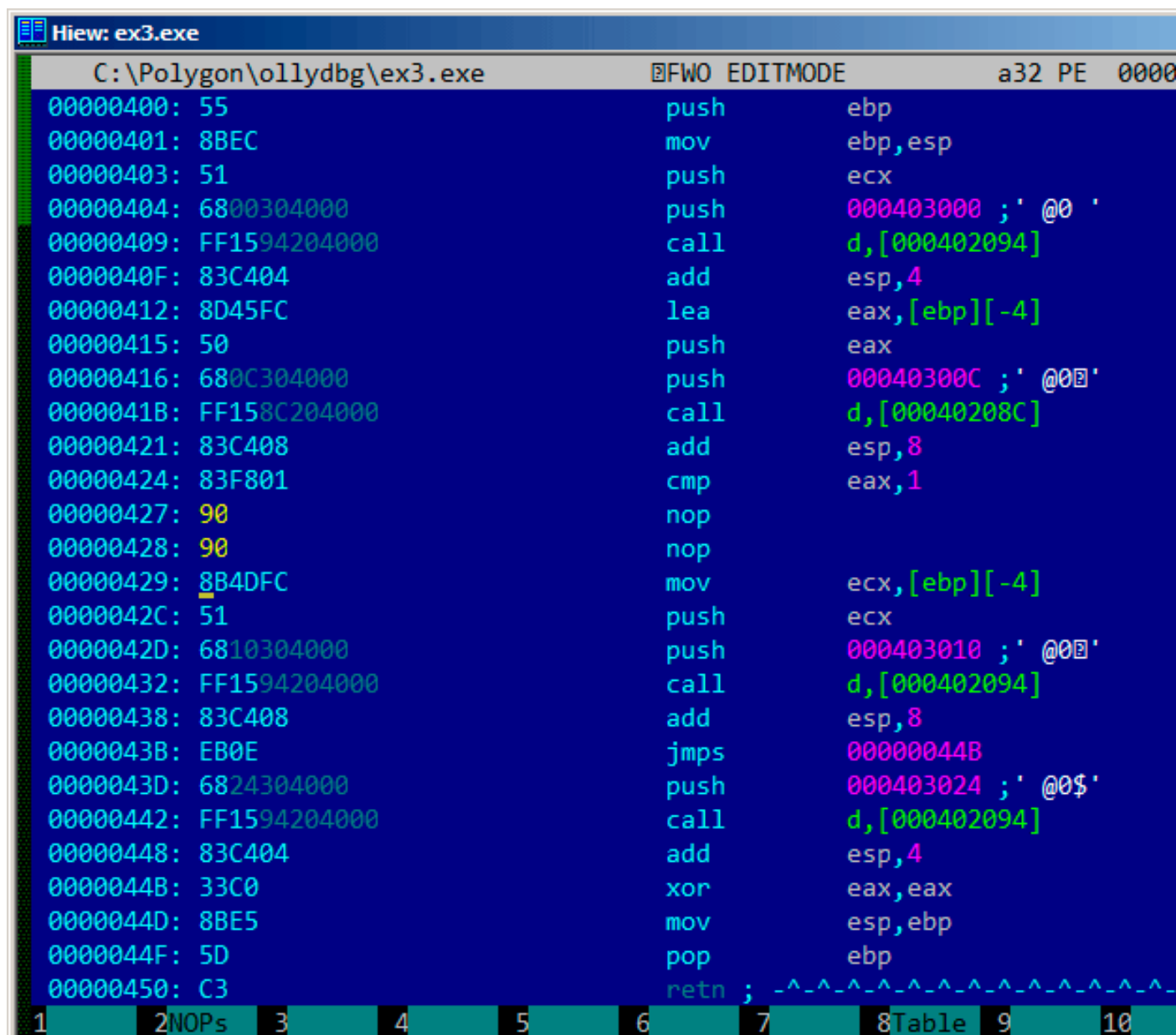
Рис. 1.22: Hiew: замена JNZ на два NOP-а
