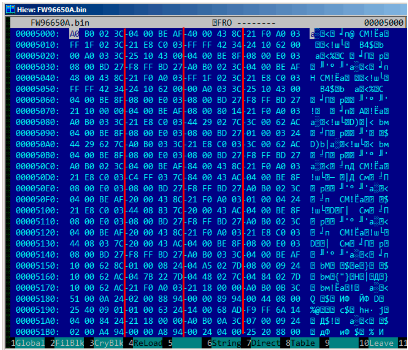
Рис. 5.9: Hiew: очень типичный код для MIPS
