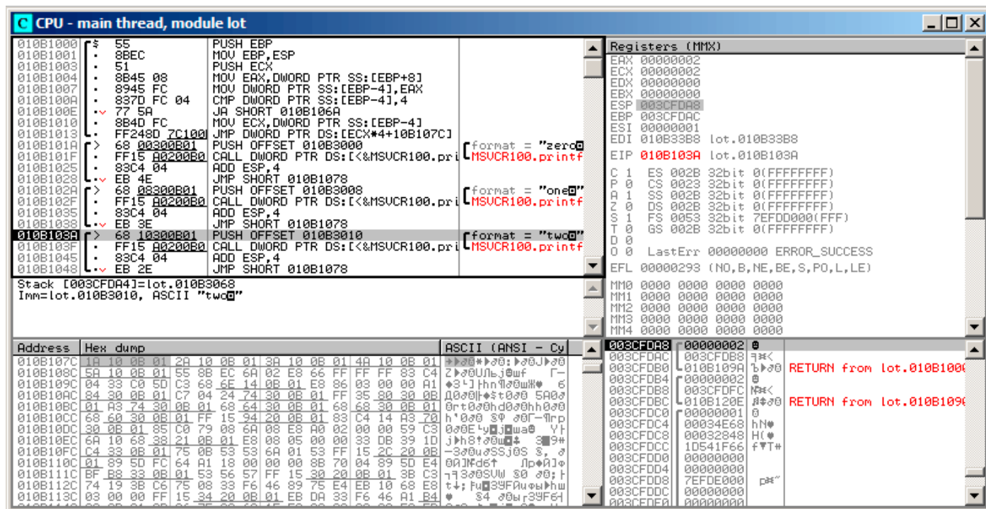
Рис. 1.45: OllyDbg: теперь мы на соответствующей метке case:
