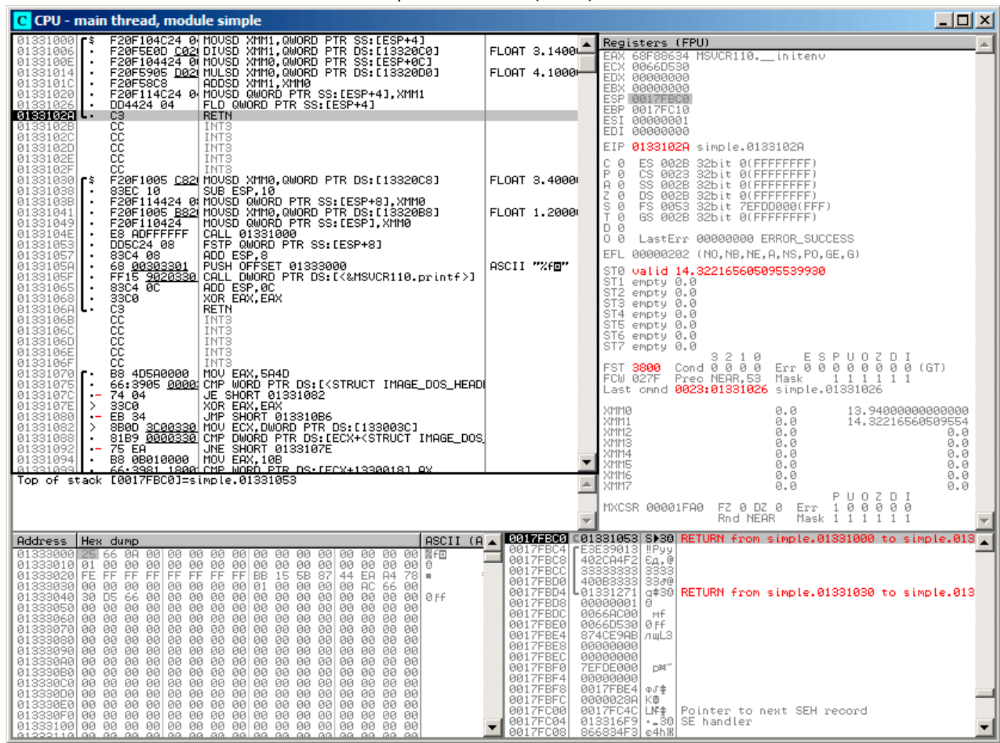
Рис. 1.109: OllyDbg: FLD оставляет результат функции в ST(0)
