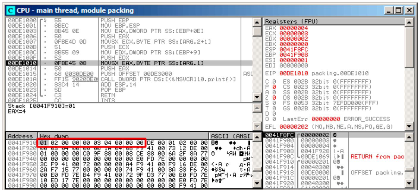
Рис. 1.98: OllyDbg: Перед исполнением printf()
