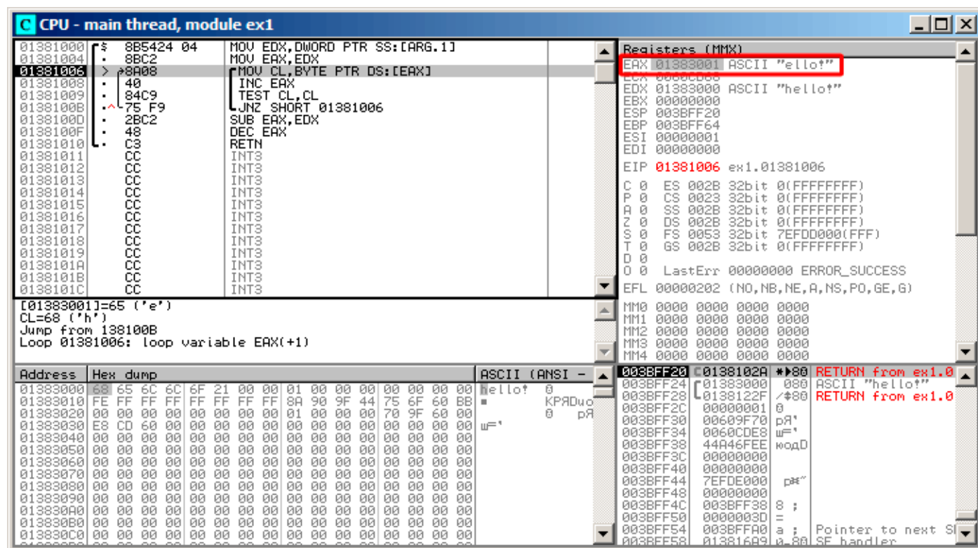
Рис. 1.51: OllyDbg: начало второй итерации
