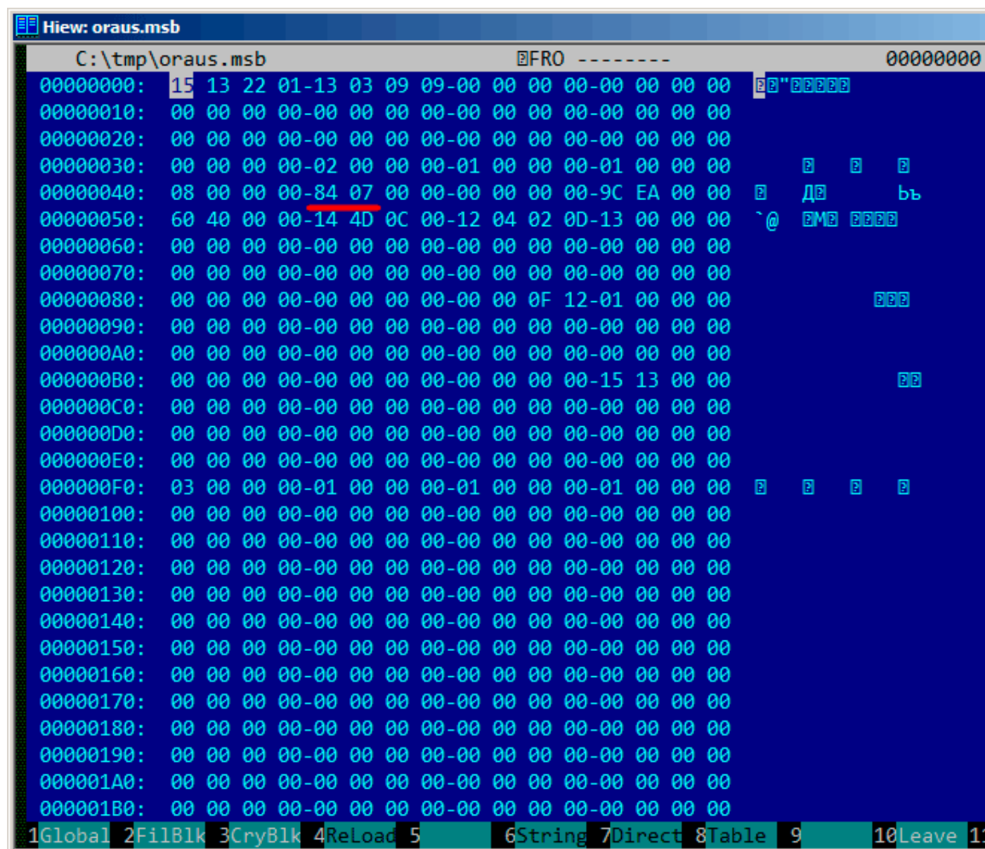
Рис. 9.28: Hiew: заголовок файла
