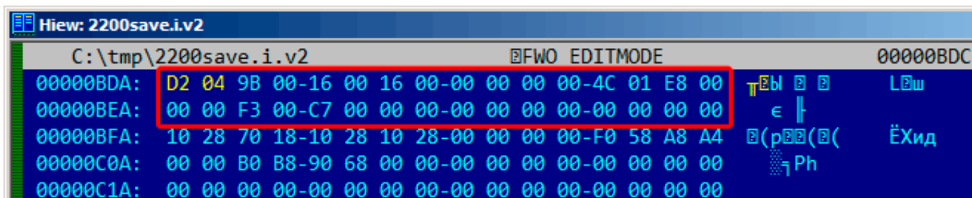
Рис. 9.16: Hiew: запишем там (0x4D2)
