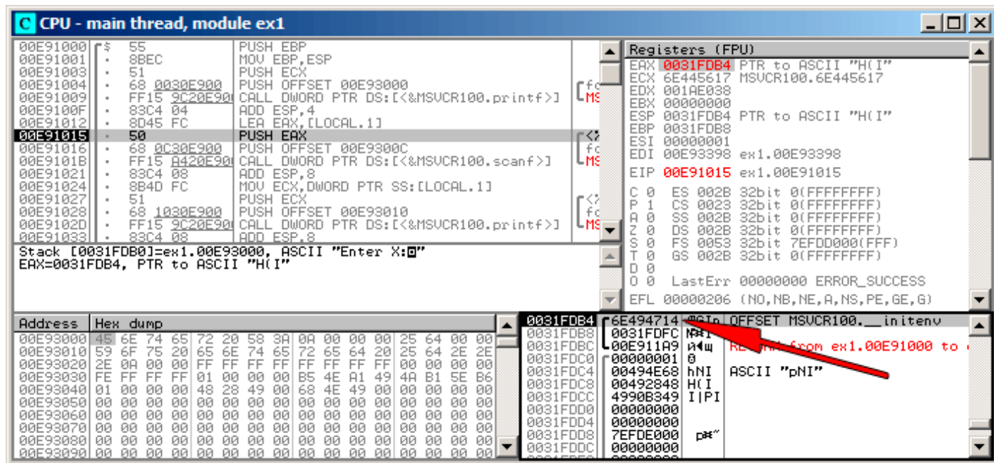
Рис. 1.12: OllyDbg: вычисляется адрес локальной переменной
