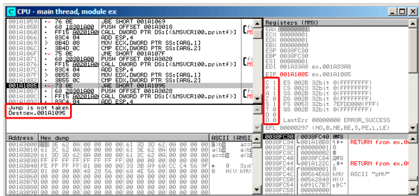
Рис. 1.28: OllyDbg: f_unsigned() : третий условный переход
