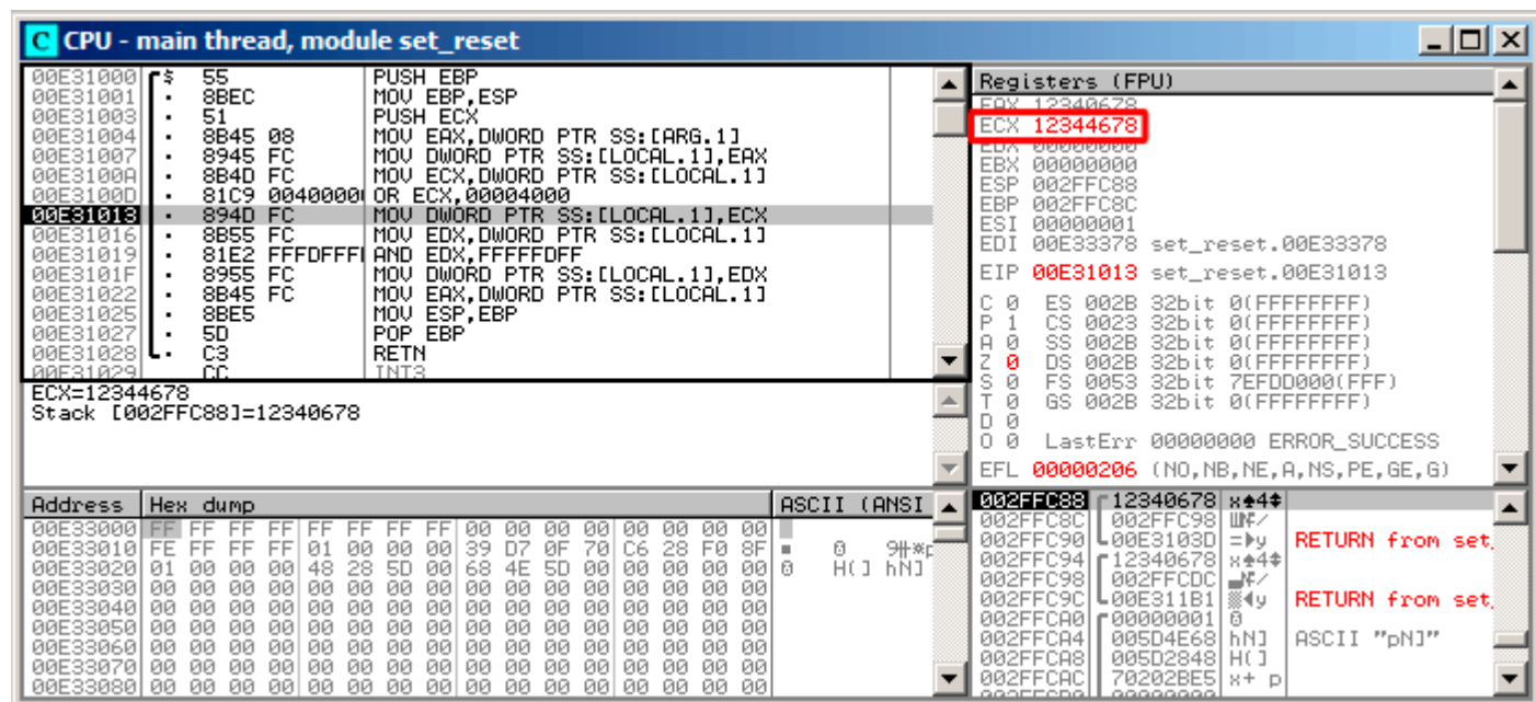
Рис. 1.87: OllyDbg: OR сработал
