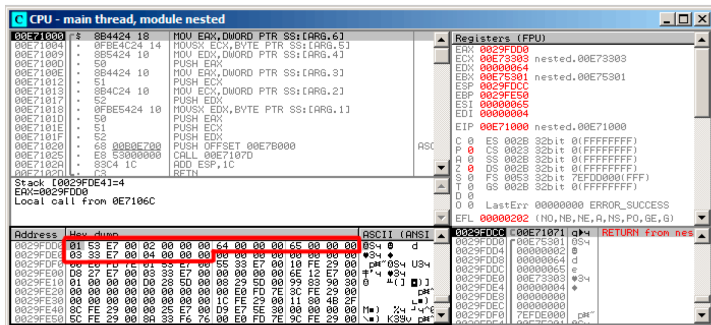
Рис. 1.99: OllyDbg: Перед исполнением printf()
