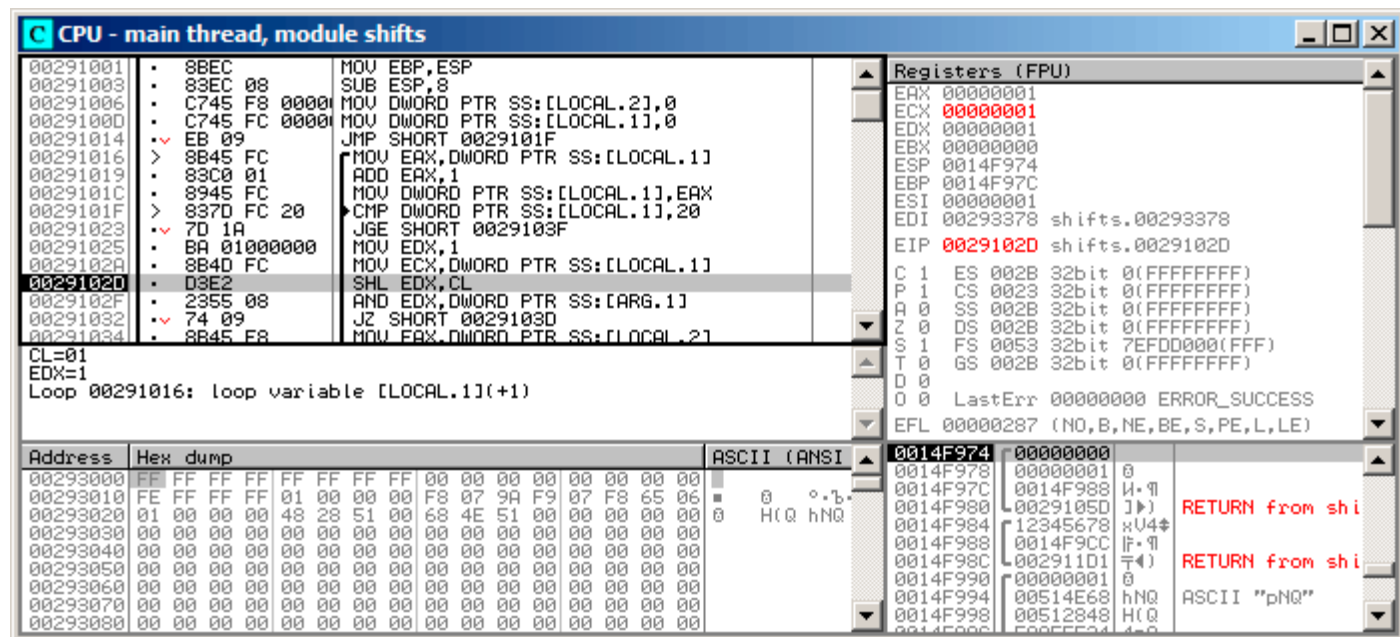
Рис. 1.90: OllyDbg: i = 1 , i загружено в ECX
