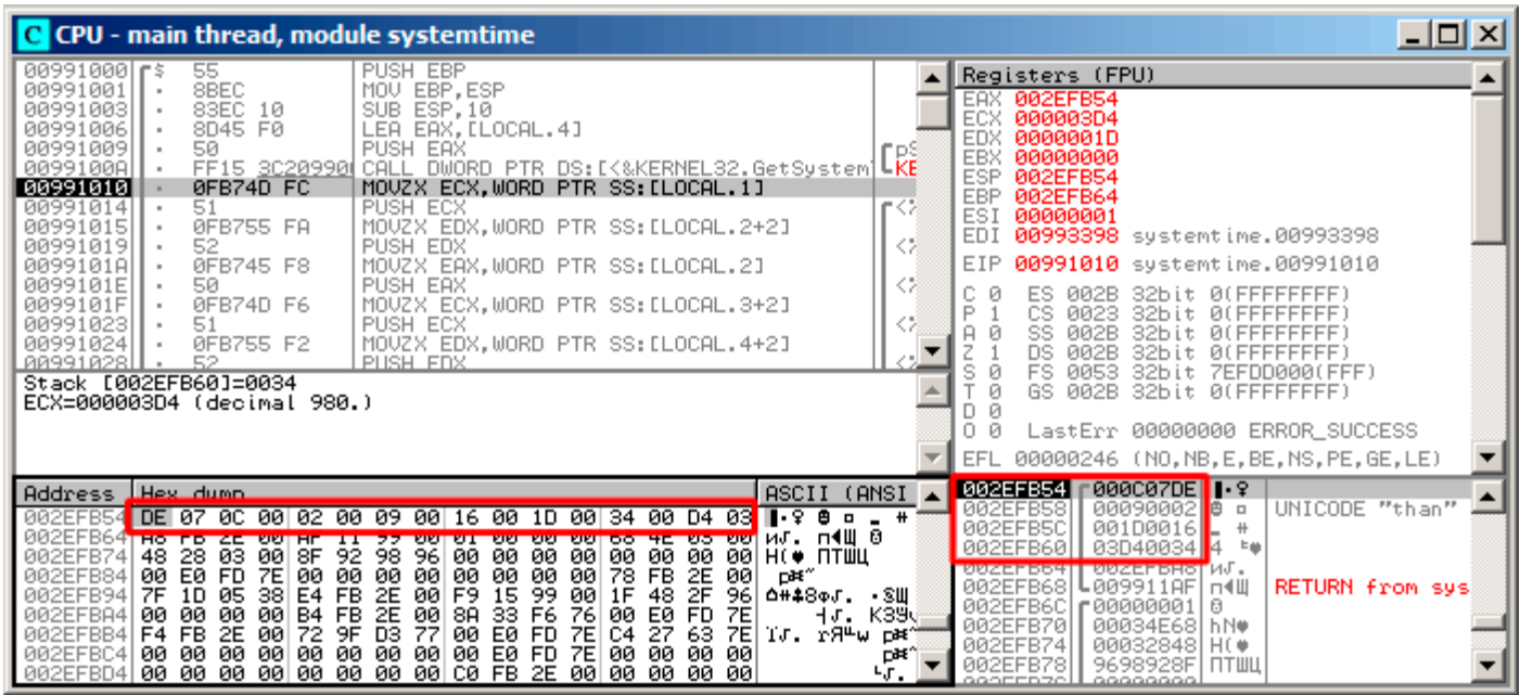
Рис. 1.96: OllyDbg: GetSystemTime() только что исполнилась
