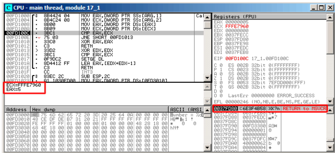
Рис. 1.103: OllyDbg: второй вызов comp()
