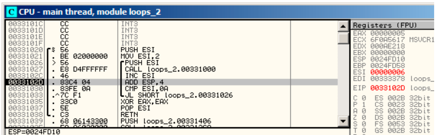
Рис. 1.47: OllyDbg: тело цикла только что отработало с i = 6
