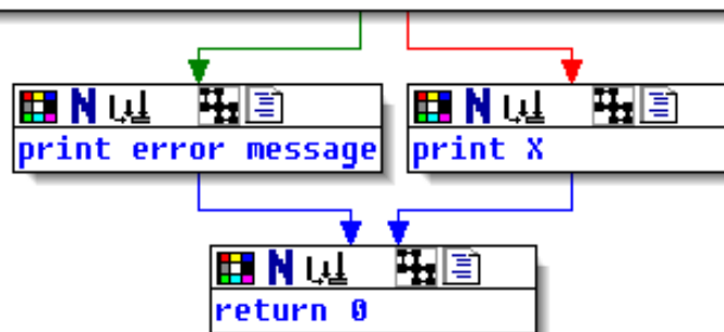
Рис. 1.18: Отображение в IDA в виде графа с тремя свернутыми блоками
