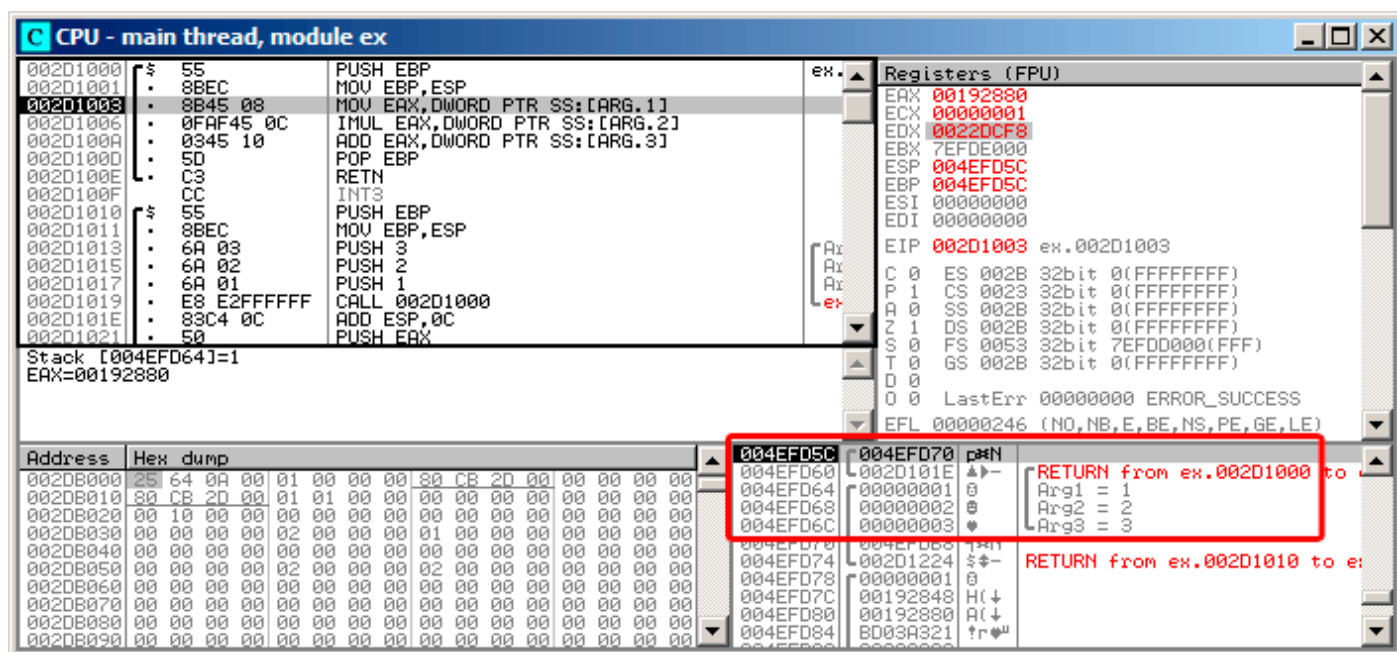
Рис. 1.23: OllyDbg: внутри функции f()
