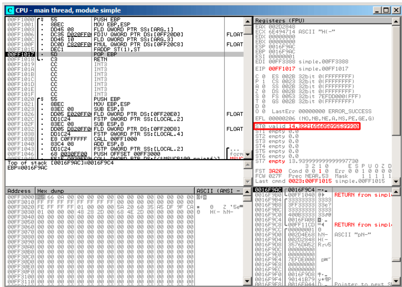
Рис. 1.58: OllyDbg: FADDP исполнилась
