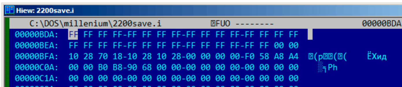
Рис. 9.18: Hiew: установим максимальные значения
